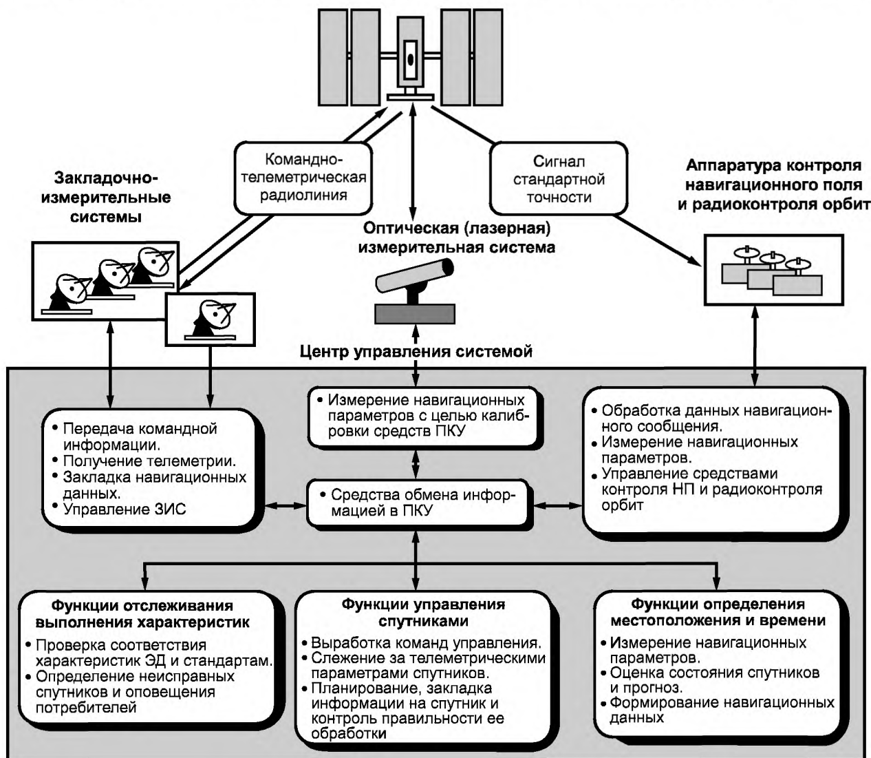
Рисунок А.2 — Процесс управления системой спутников
