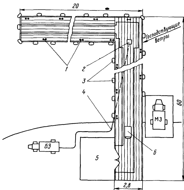
Рис. 3 Пирс: 1 — кнехты, 2 — колодец для раздаточного устройства, 3 — автопокрышки, 4 — топливопровод; 5 — склад отдела перевозок; 6 — загрузочная тележка
