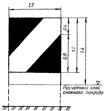
Рис. 3.23. Знак боковых границ КРБ
