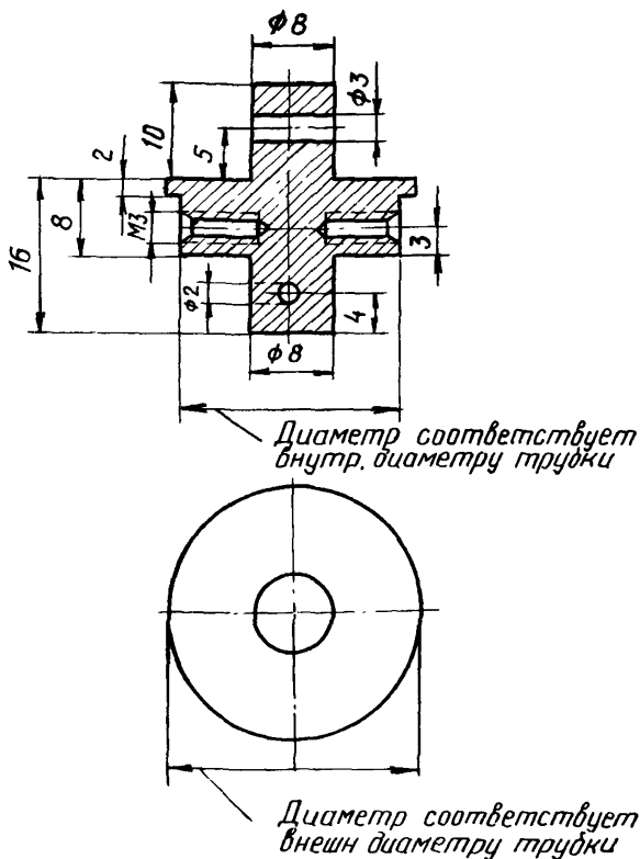
Рис 5. Втулка (2).
