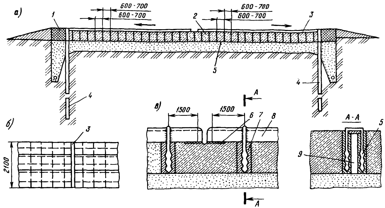
Рис. 4.5. Заземляющее устройство:
