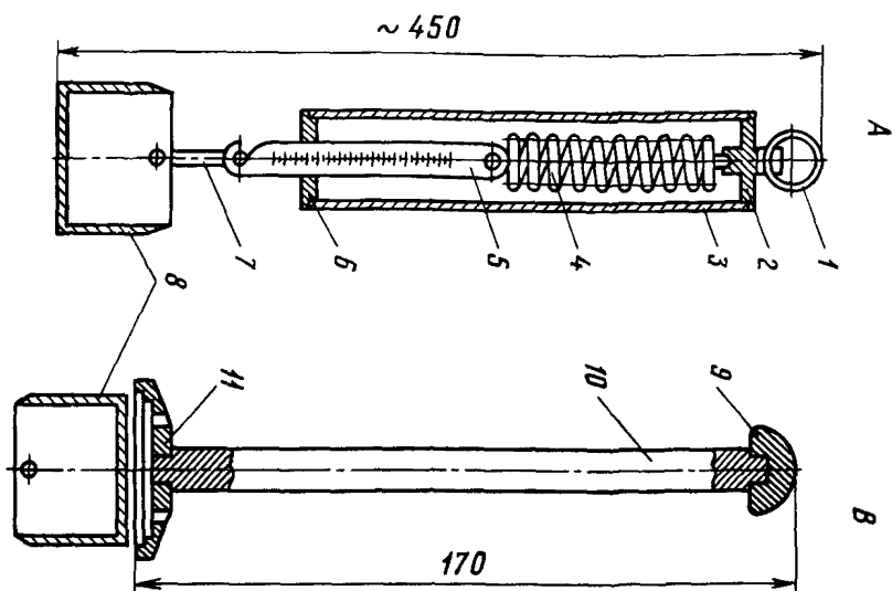
Рис. 4. Пружинный плотномер:
