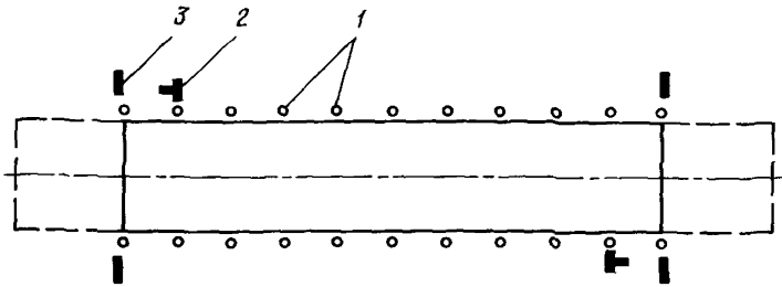
Рис 3 17 Схема оборудования маркировочными знаками аэродромов класса E и неклассифицированных.
