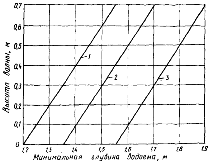
График для определения минимальной глубины водоема ( H_{\min} ) при эксплуатации самолета Ан-2В: 1 — дно из слабых мягких грунтов; 2 — дно из плотных песков и глин; 3 — дно из неразмываемых плотных грунтов
