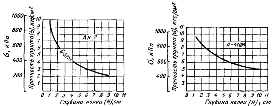
Рис. 6а. Графики зависимости прочности грунта от глубины колеи для самолетов Ан-2 и Л-410М
