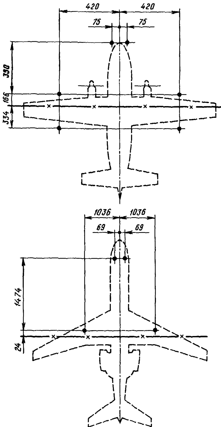
Рис 4 Зд. Схема расположения на покрытии точек швартовки самолетов: 1 — Л-410, Л-410 УВП; 2 — Як-42 — — — — — X — — — — — ось основных опор самолета
