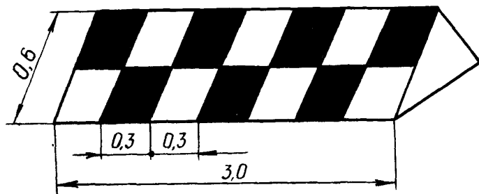
Рис 3.29 Знак для обозначения опасных мест
