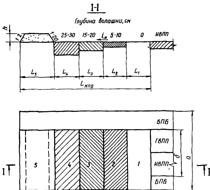
Рис. 47 Схема грунтовой тормозной площадки: a — ширина летной полосы, b — ширина рабочей площадки; L_{кпб} — длина концевой полосы безопасности; L_1, L_2, L_3, L_4, L_5 — длины участков тормозной площадки; 2 — 4 — вспашанные на различную глубину и заборонированные участки концевой полосы безопасности, 5 — песчаная насыпь
