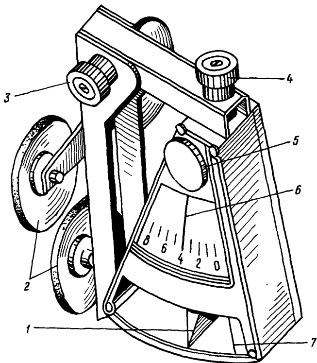
Рис 3. Деселерометр:
