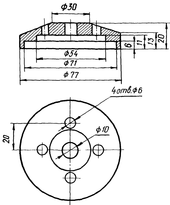
Рис. 12. Опорная площадка (11).
