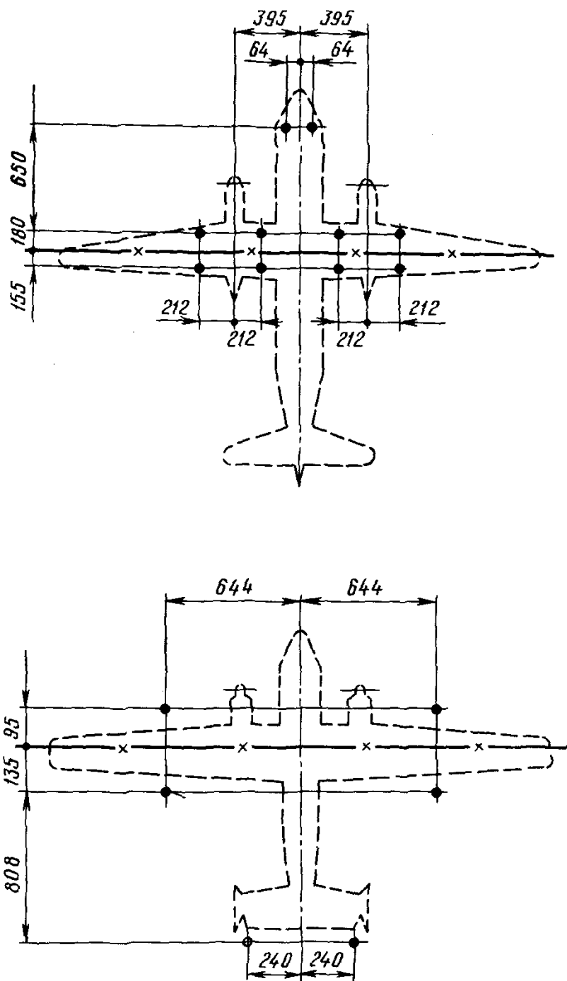
Рис. 4.36. Схема расположения на покрытии точек швартовки самолетов: 1 — Ан-24, Ан-26, Ан-30; 2 — Ан-28 — — — — — × — — — — — ось основных опор самолета
