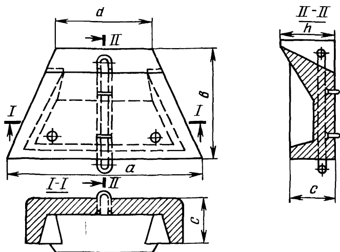
Рис. 2 Якорь типа «лягушка»
