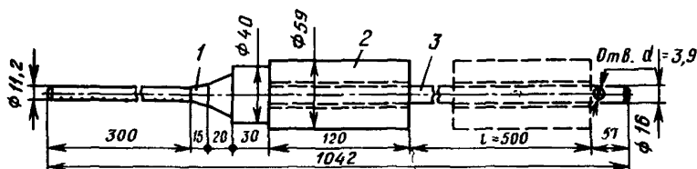
Рис. 1. Ударник У-1: 1 — наконечник; 2 — груз (гиря), 3 — направляющий шток
