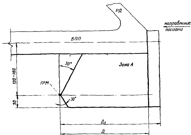
Рис. 2.4. Зоны глиссадных радиомаяков СП-75, СП-80 Н. Примечание. «Д» определяется в соответствии с ВСН 7—86
