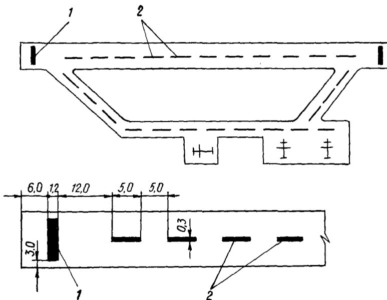
Рис. 3.5. Маркировка ИВП неклассифицированных аэродромов: 1 — порог; 2 — ось ИВП
