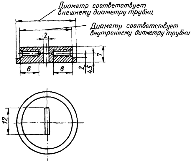
Рис 8 Направляющая шкала (6)
