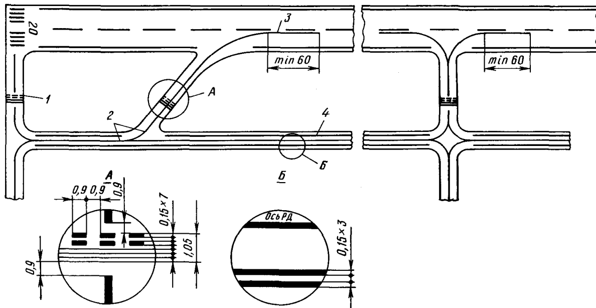
Рис. 3.6. Маркировка РД: 1 — место ожидания самолетов; 2 — ось РД; 3 — участок сопряжения РД с ИВПП; 4 — рулевая боковая маркировочная полоса
