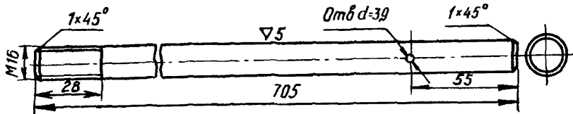
Рис 4 Шток направляющий
