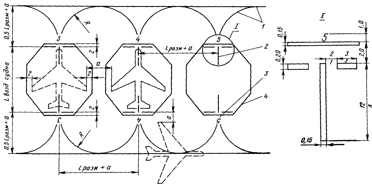
Рис 3.7. Маркировка МС:
