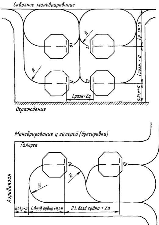
Рис 3.8 Маркировка перрона
