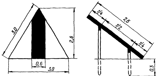
Рис 3.25 Знак подхода
