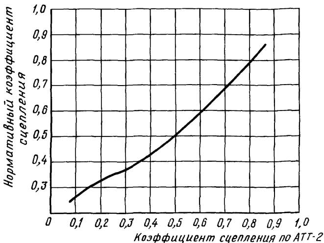
Рис 2. Корреляционный график
