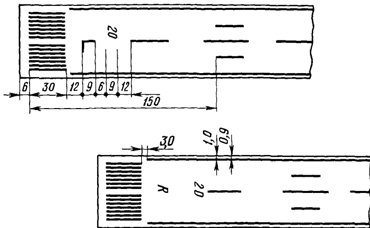
Рис. 3.4 Маркировка параллельных ИВП: L — левая; R — правая
