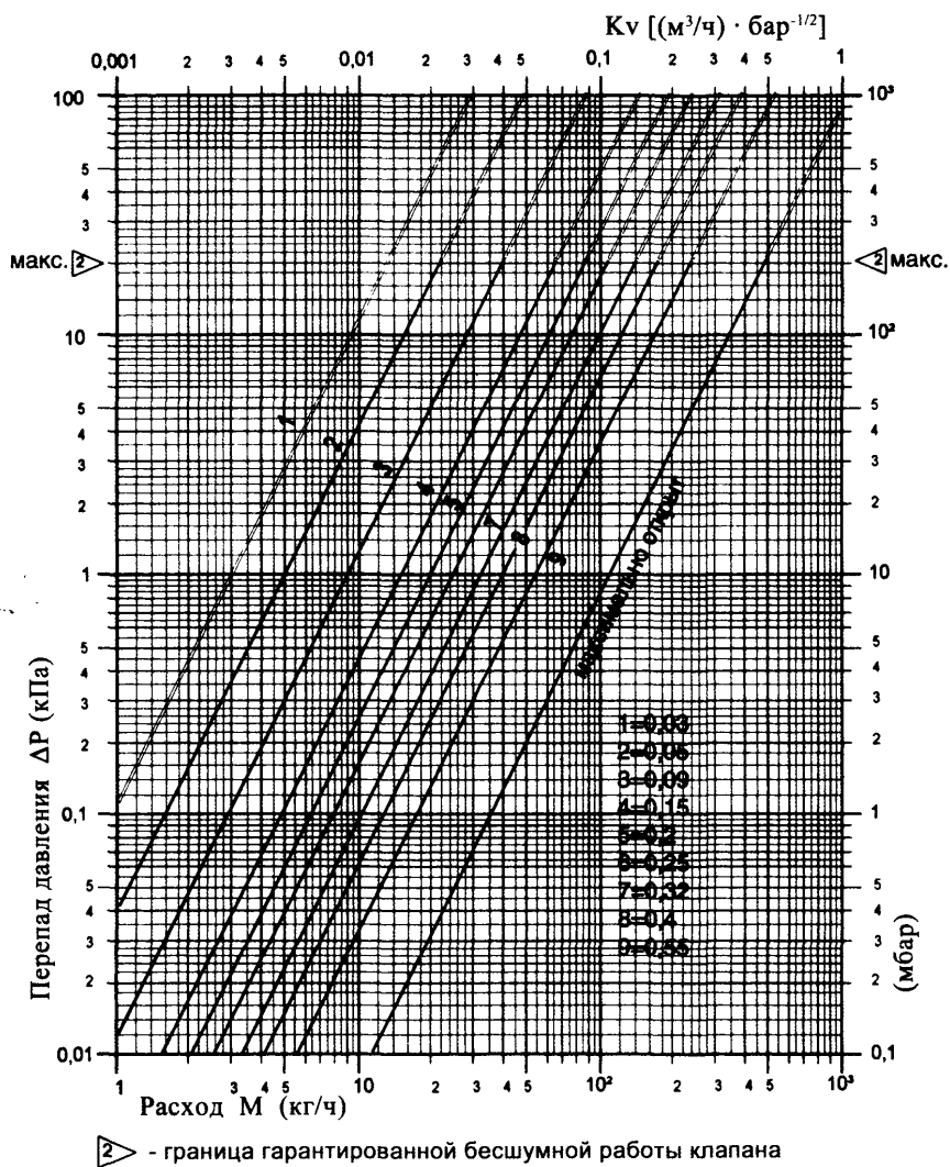
Рис. 3.1. Гидравлические характеристики термостатов «ГЕРЦ-TS-90-V» с присоединительными размерами 3/8" и 1/2" с настройкой на режим 2K (2°C) и при снятой термостатической головке (при полном открытии вентиля)
