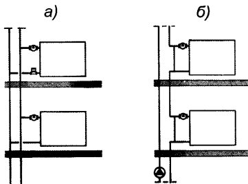
Рис. 2.2. Схемы вертикальных систем отопления с радиаторами «Zehnder Charleston» а – двухтрубная, б – однотрубная
