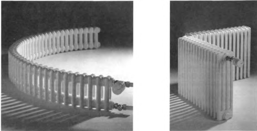
Рис. 2.6. Общий вид радиатора «Zehnder Charleston» полукруглой формы и радиатора «Zehnder Charleston Completto» угловой конфигурации
