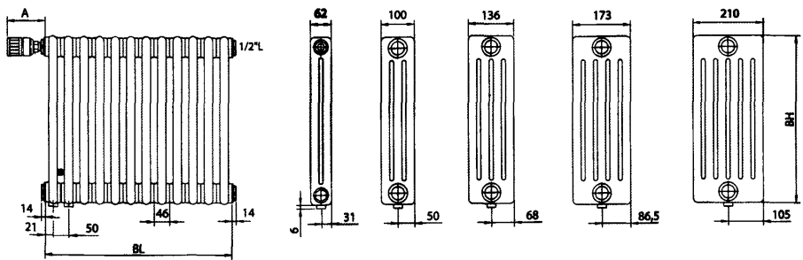
Рис. 1.3. Номенклатурный ряд радиаторов «Zehnder Charleston Completo»
