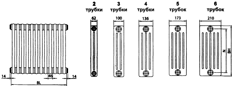
Рис. 1.2. Номенклатурный ряд радиаторов «Zehnder Charleston»
