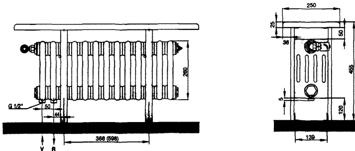
Рис. 1.7. Радиатор-скамейка «Zehnder Charleston Relax» модели CR 5026-13
