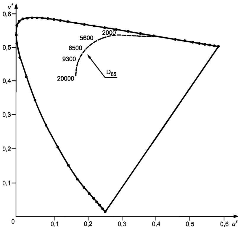
Рисунок 2 — Положение иллиуминанта МКО D 65 и цветных температур на равноконтрастном цветовом графике МКО 1976 г.
