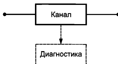
Рисунок В.3 — Структурная схема архитектуры 1oo1
