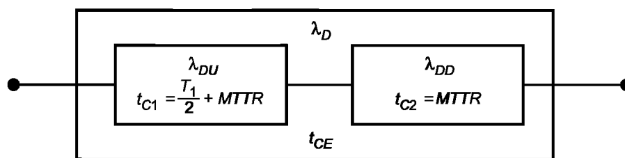
Рисунок В.4 — Схема расчета надежности архитектуры 1oo1
