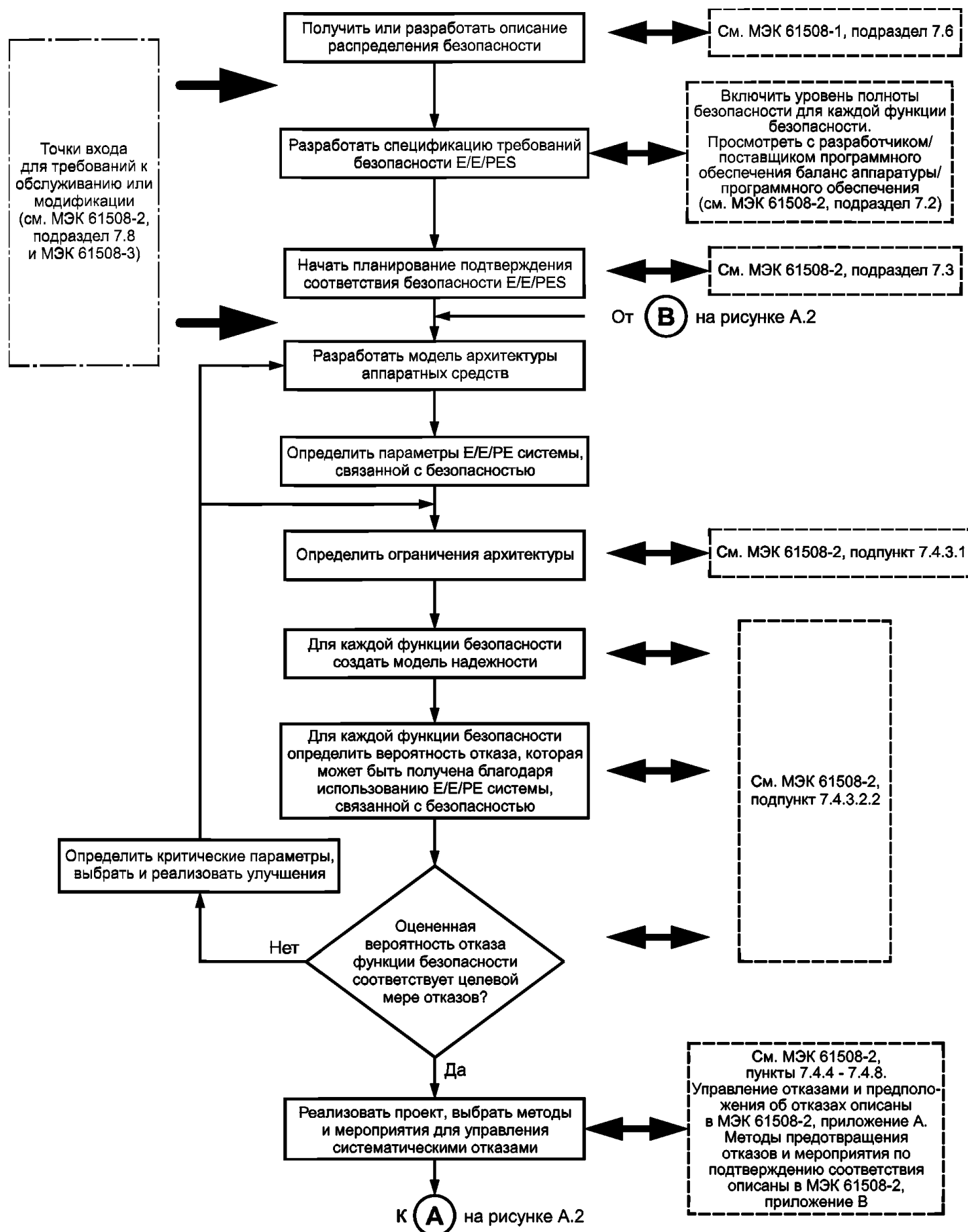
Рисунок А.1 — Функциональные этапы применения МЭК 61508-2
