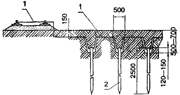
Рисунок 7 — Соединение заземлителей
