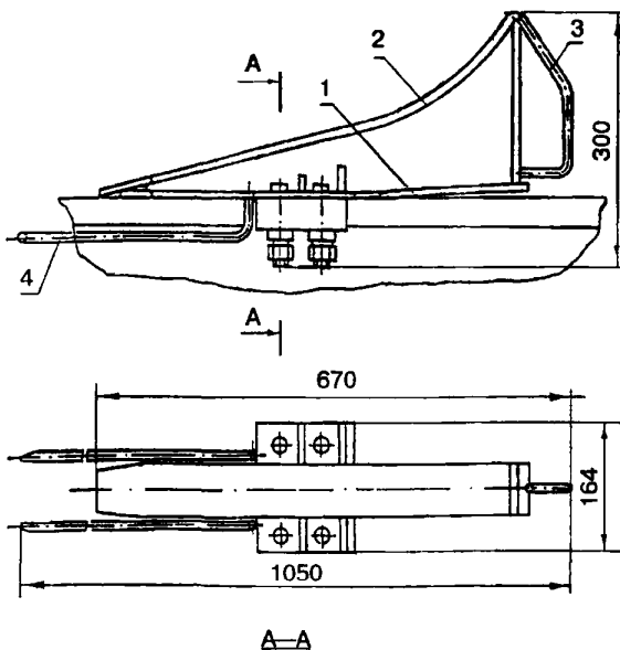
Рисунок 5 — Крепление тупикового упора к рельсу
