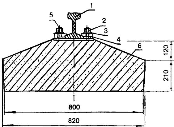
Рисунок 4 — Крепление рельса к балке
