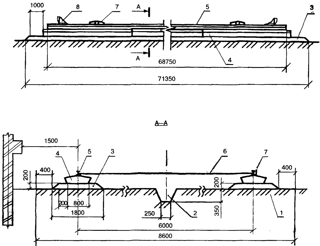
Рисунок 1 – Рельсовый путь башенного крана
