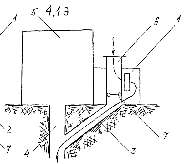
Рис. 4.1. Основные схемы компоновки калориферных установок
