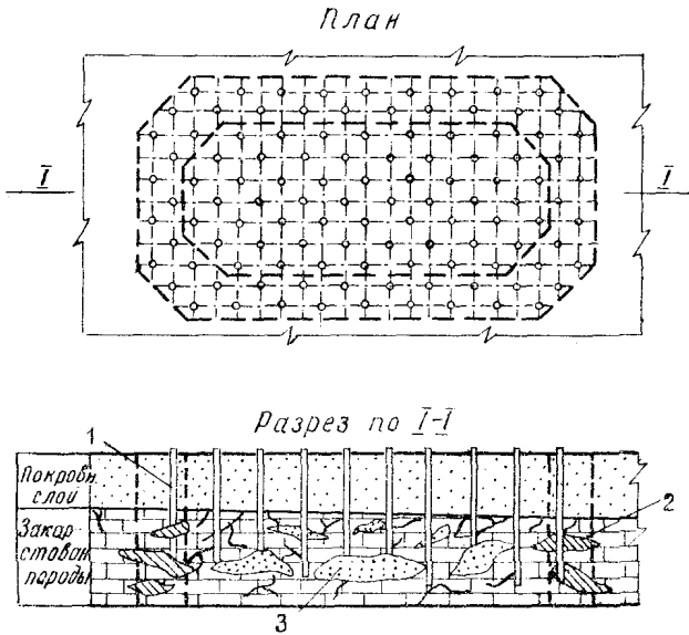
Рис. 2. Схема закрепления карстового участка комбинированным тампонируанием
