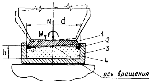
Рис. 8. Схема шаровой опоры
