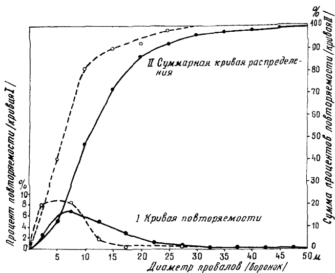
Рис. I. График распределения карстовых провалов и воронок по величине их диаметров (район г. Дзержинска)
