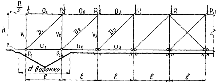
Рис. 6. Схема применения дополнительных связей в каркасе промздания
