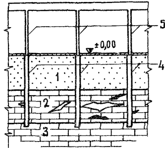
Рис. 4. Схема фундаментов из буровых опор глубокого заложения или из свай-стоек
