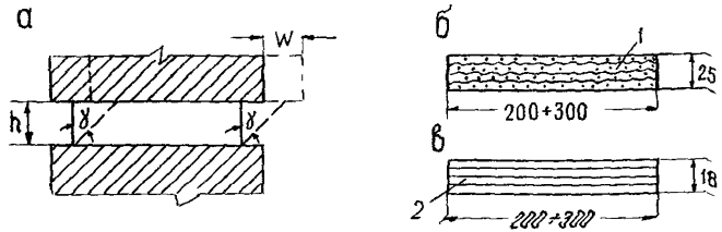
Рис. 7. Резиновая подвижная опора
