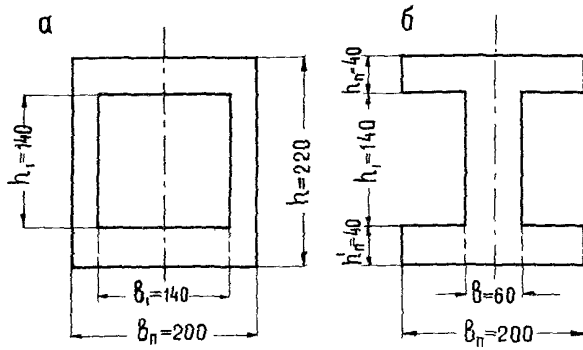
Рис. 13. Поперечные сечения балочного фундамента а - действительное; б - эквивалентное.
