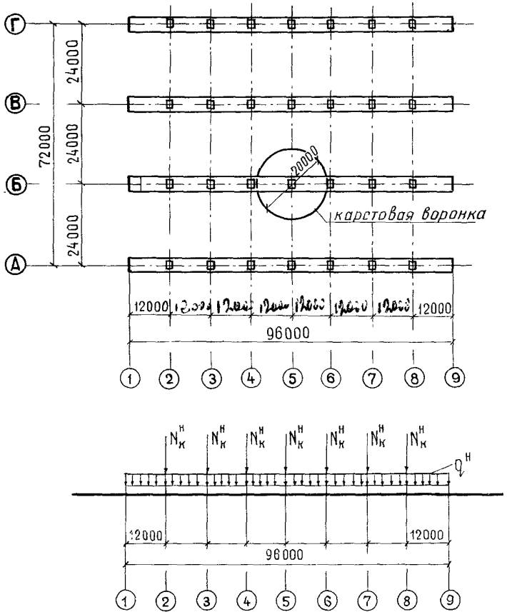
Рис. 12. План фундаментов и расчетная схема балки на сплошном у ругом основании
