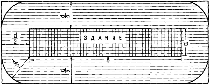
Рис. 10. Схема параметров "зоны поражения" здания карстовыми провалами
