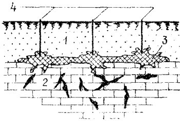
Рис. 3. Схема закрепления несвязных грунтов, покрывающих закарстованные породы
