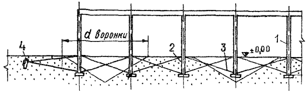
Рис. 5. Схема фундамента с подпругами
