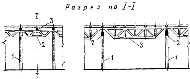
Рис. 9. Схема покрытия здания
