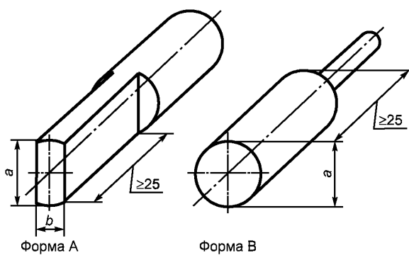
Рисунок 2 — Щупы формы А и В (см. 8.2.4.5.2 и таблицу 7)
