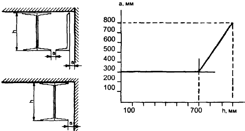
Рисунок 1 – Минимально разрешенное расстояние между элементами конструкций (ИСО 12944-3)
