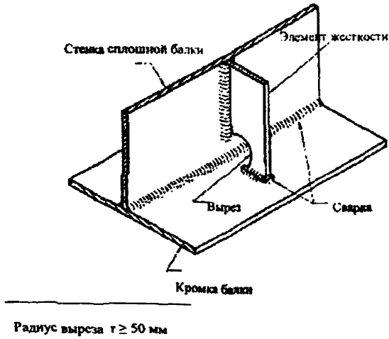
Рисунок 4 – Пример конструкции с вырезкой (ИСО 12944-3)
