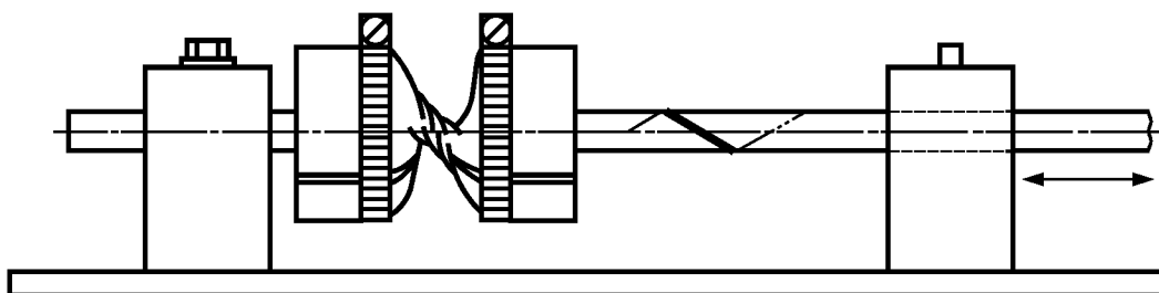
с) Полностью сжатый образец
