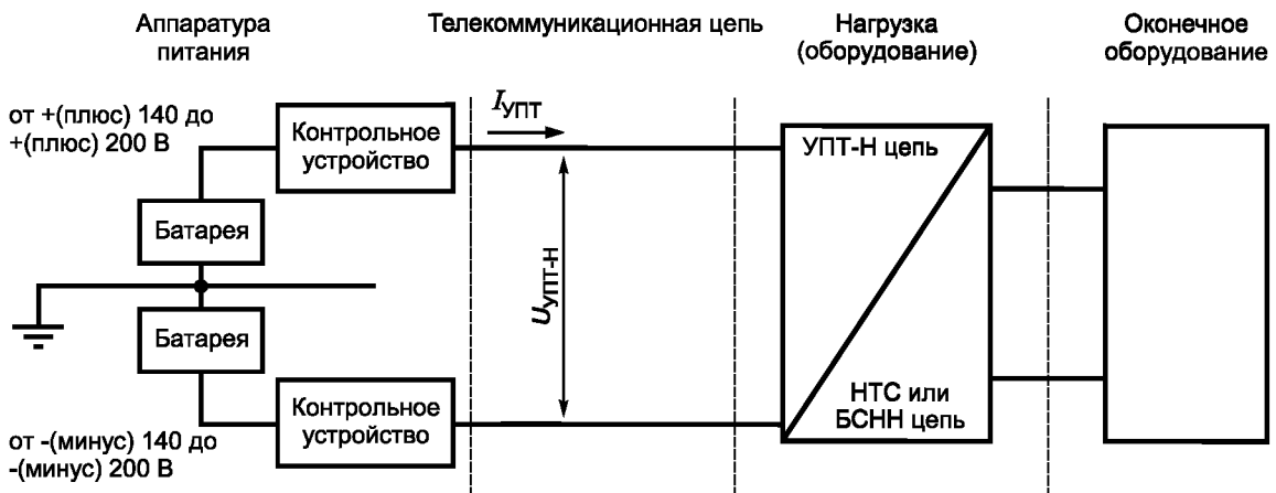
Рисунок А.2 — Пример УПТ-Н системы удаленного электропитания
