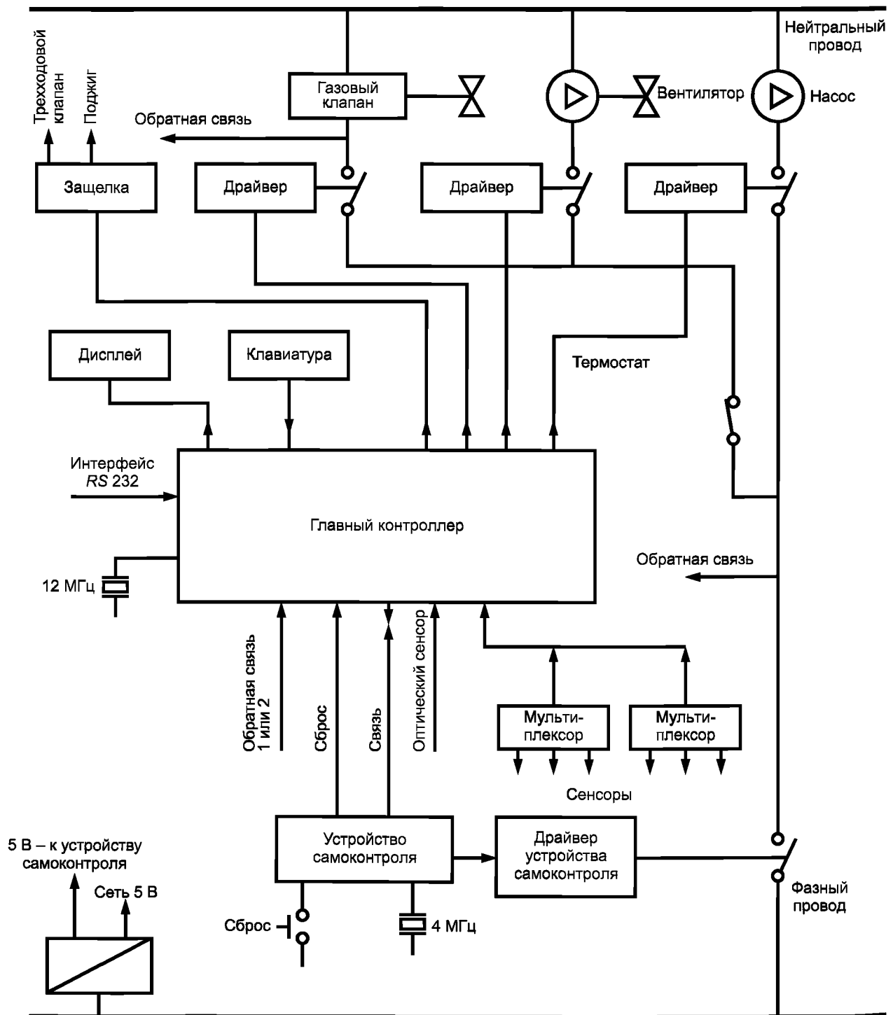
Рисунок Б.2 — Контроллер газовой горелки: структура
