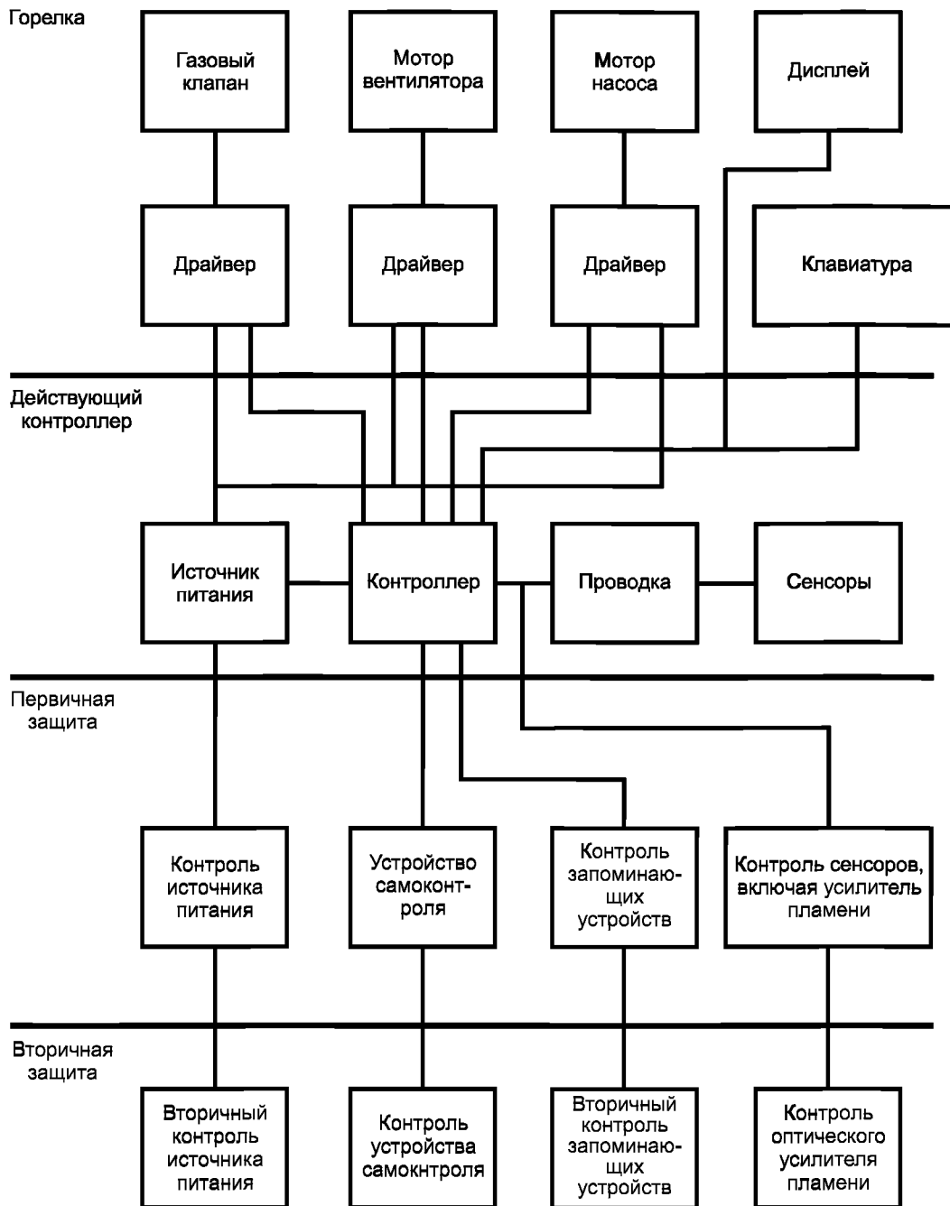
Рисунок Б.3 — Контроллер газовой горелки: блок-схема
