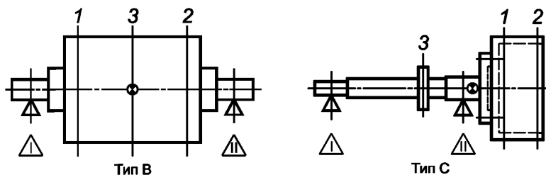
б) Горизонтальный балансировочный станок
