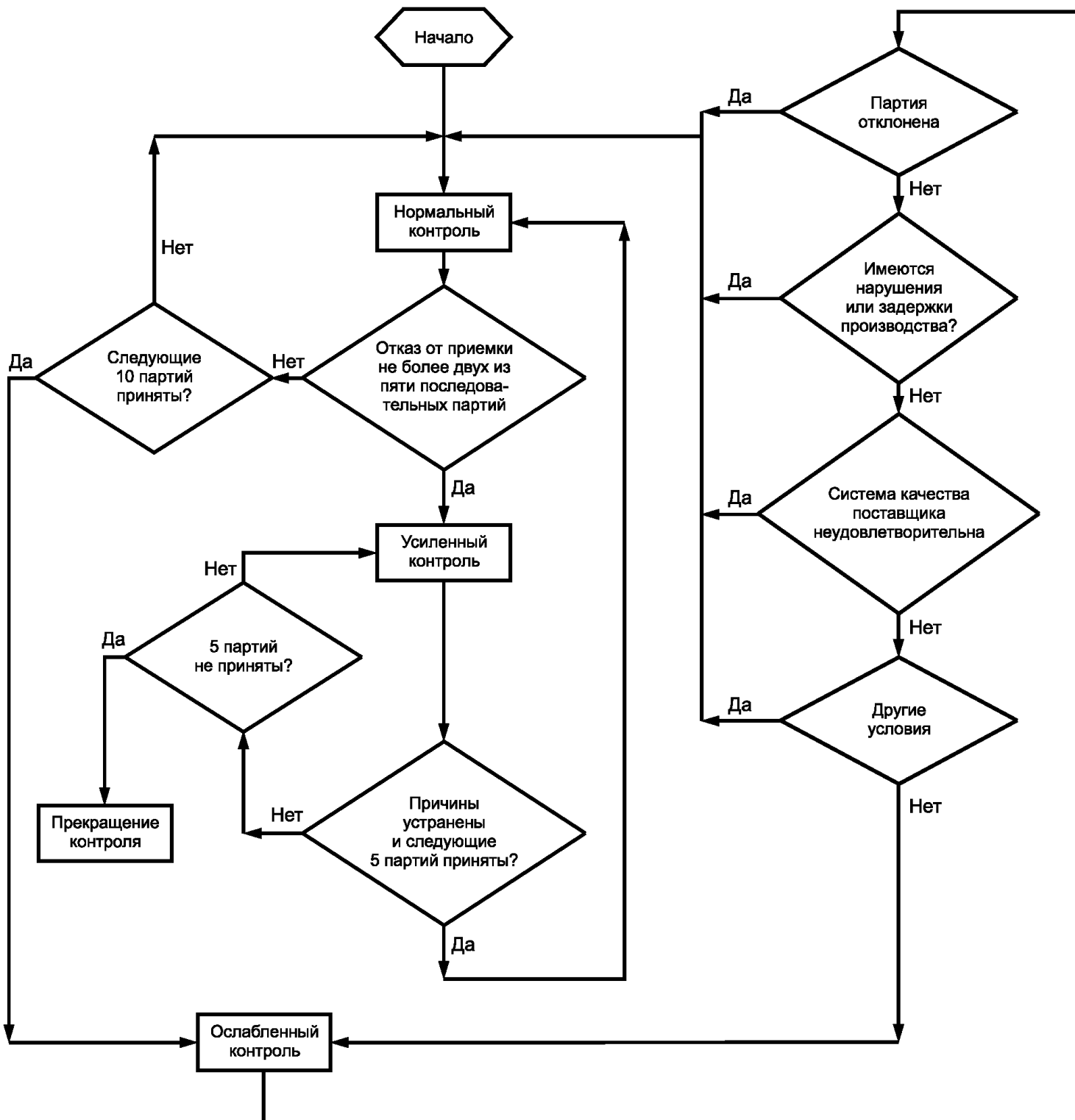
Рисунок С.1 — Процедуры переключения выборочного контроля
