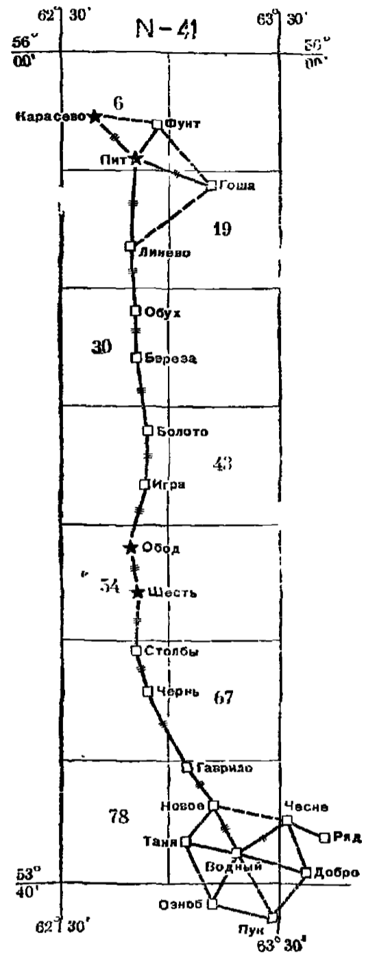
Схема звена полигонометрии 1 класса Карасево — водный
