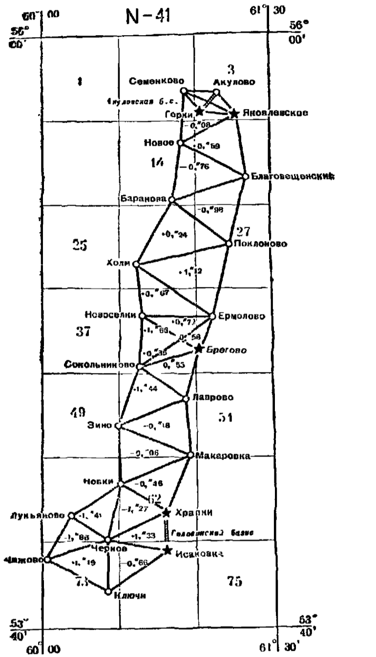
Схема звена триангуляции 1 класса Акулово — Головино
