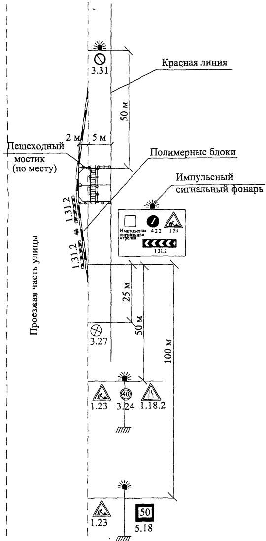
Рисунок 3- Схема организации движения.
