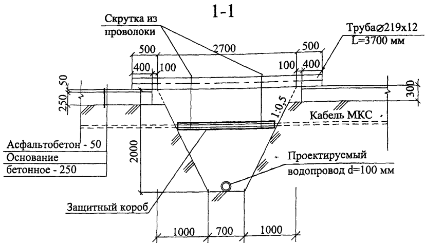
Рисунок 2- Габаритные размеры котлована.
