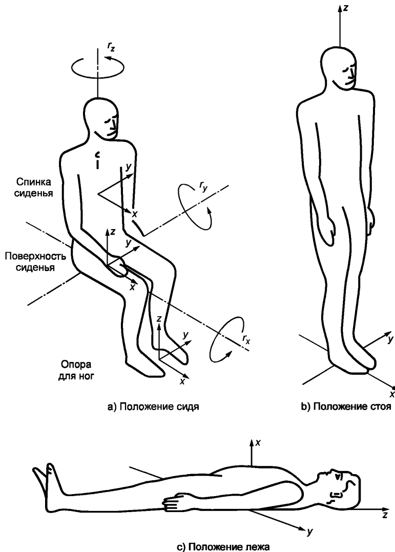
Рисунок 1 — Базицентрическая система координат для тела человека
