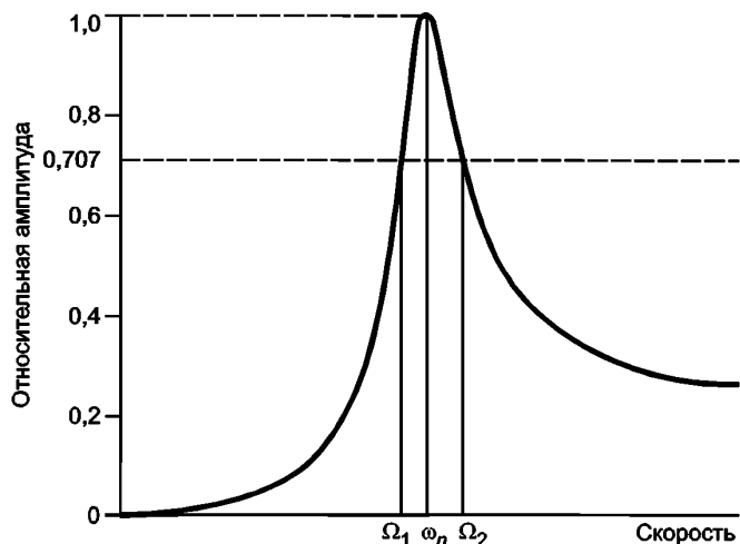
Рисунок 5 — Диаграмма Бодe для оценки модальной чувствительности
