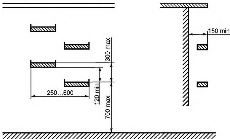
Рисунок 7 — Другие средства доступа и места обслуживания
