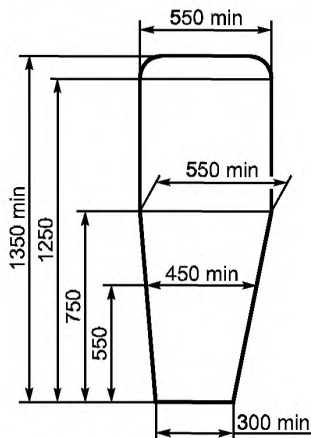
Рисунок 5 — Основные размеры дверного проема
