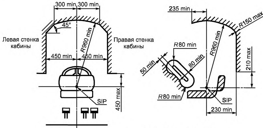
Рисунок 6 — Размеры внутреннего рабочего пространства
