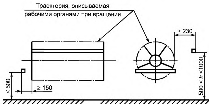
Рисунок 11 — Вращающееся подающее устройство
