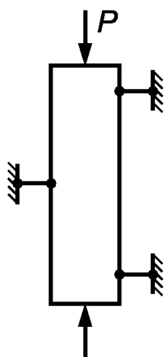
Рисунок 13 — Схемы закрепления стоек при испытании
