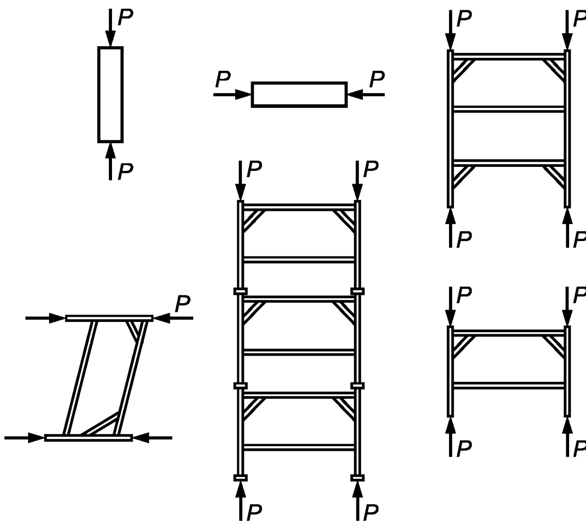
Рисунок 12 — Схемы испытания рам
