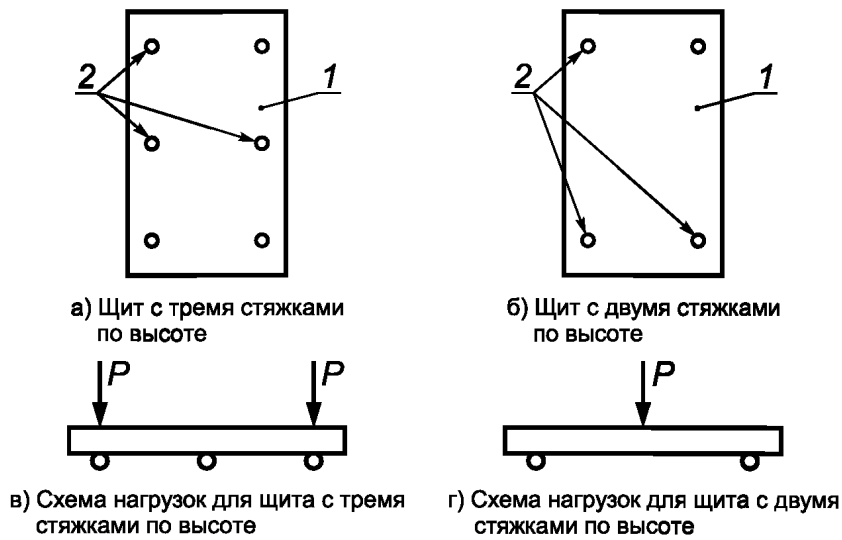
1 — щит; 2 — опора
