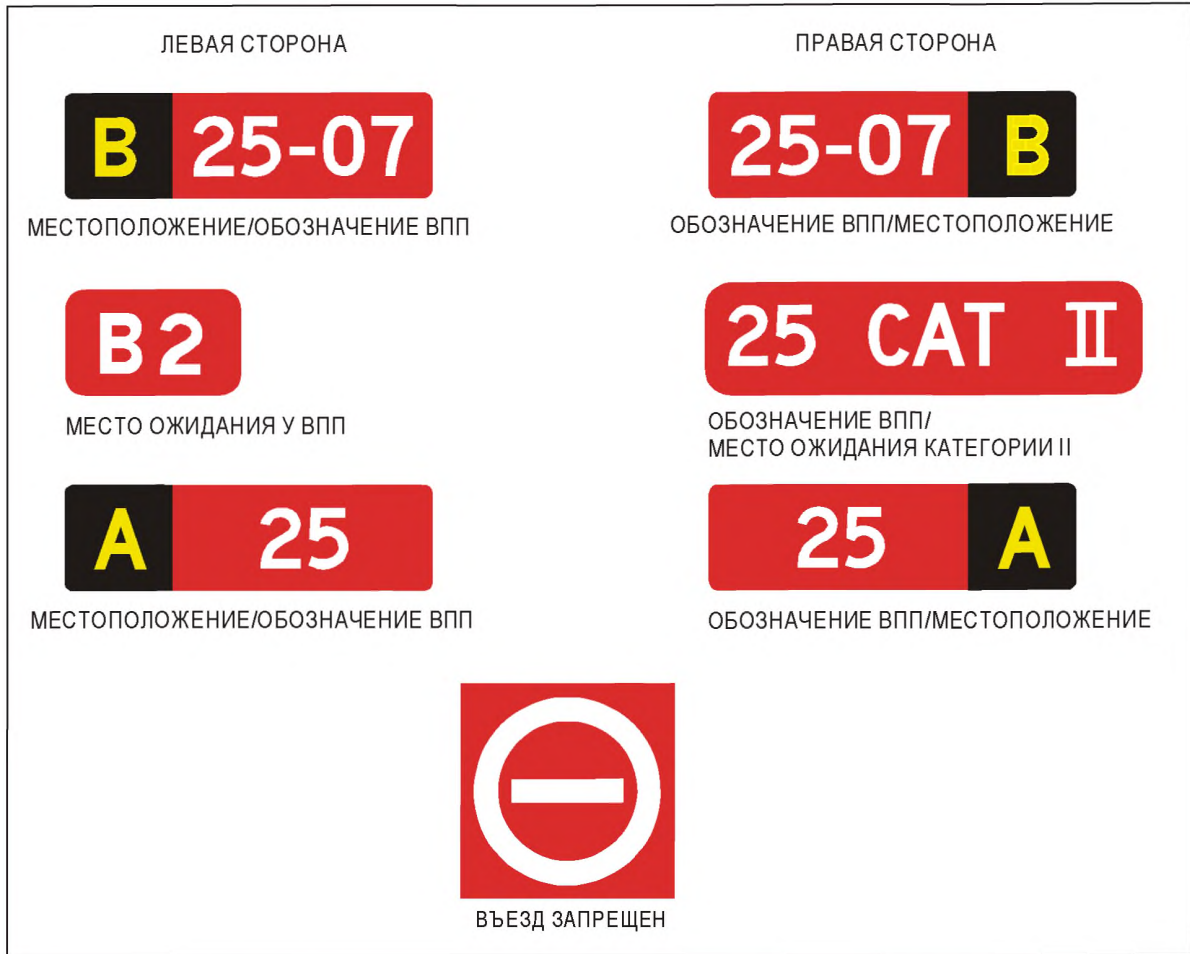
Рис. 5-30. Знаки, содержащие обязательные для исполнения инструкции
