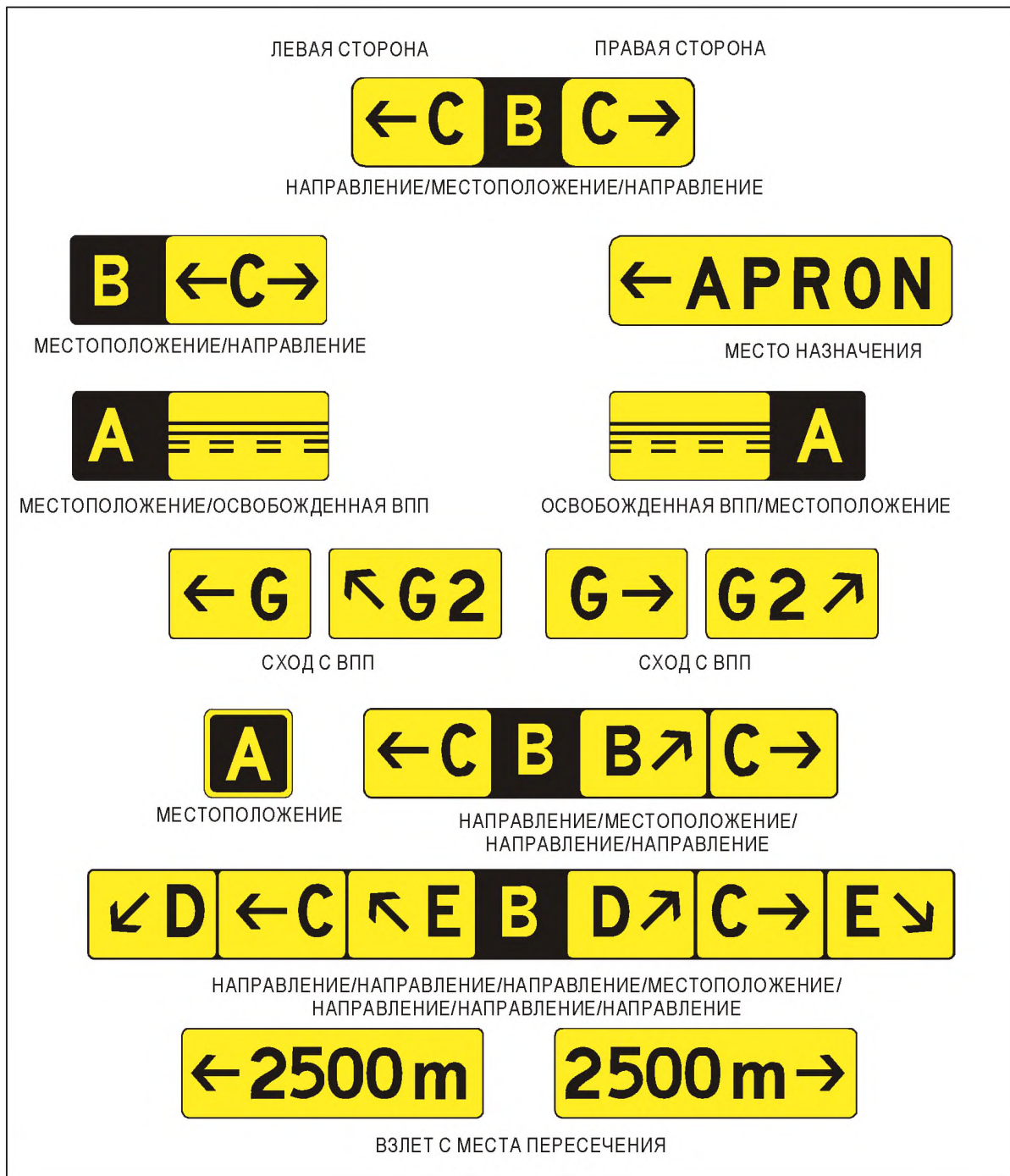
Рис. 5-31. Указательные знаки
