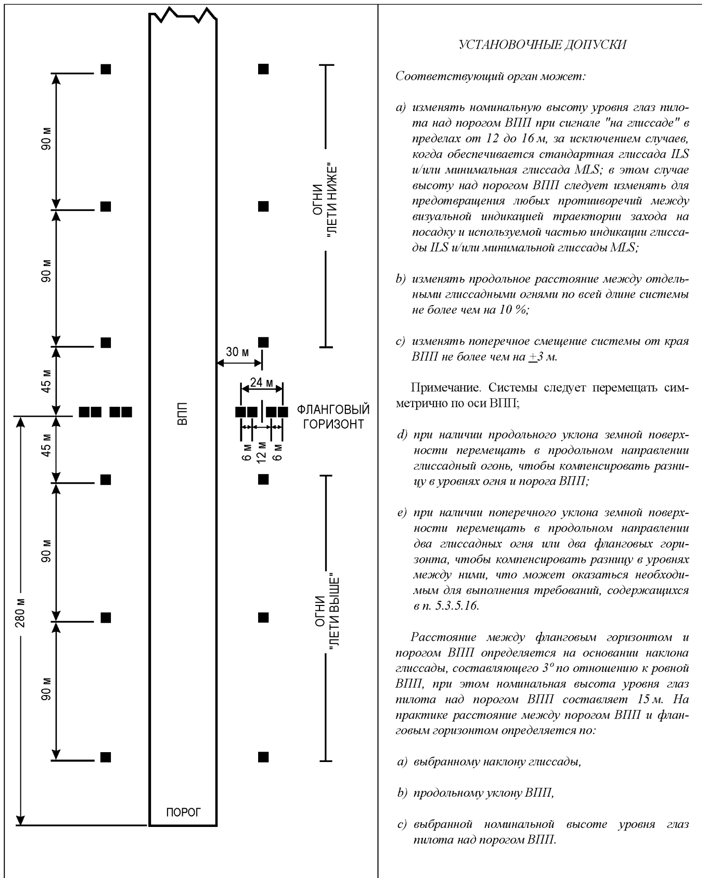
Рис. 5-17. Местоположение глиссадных огней системы T-VASIS
