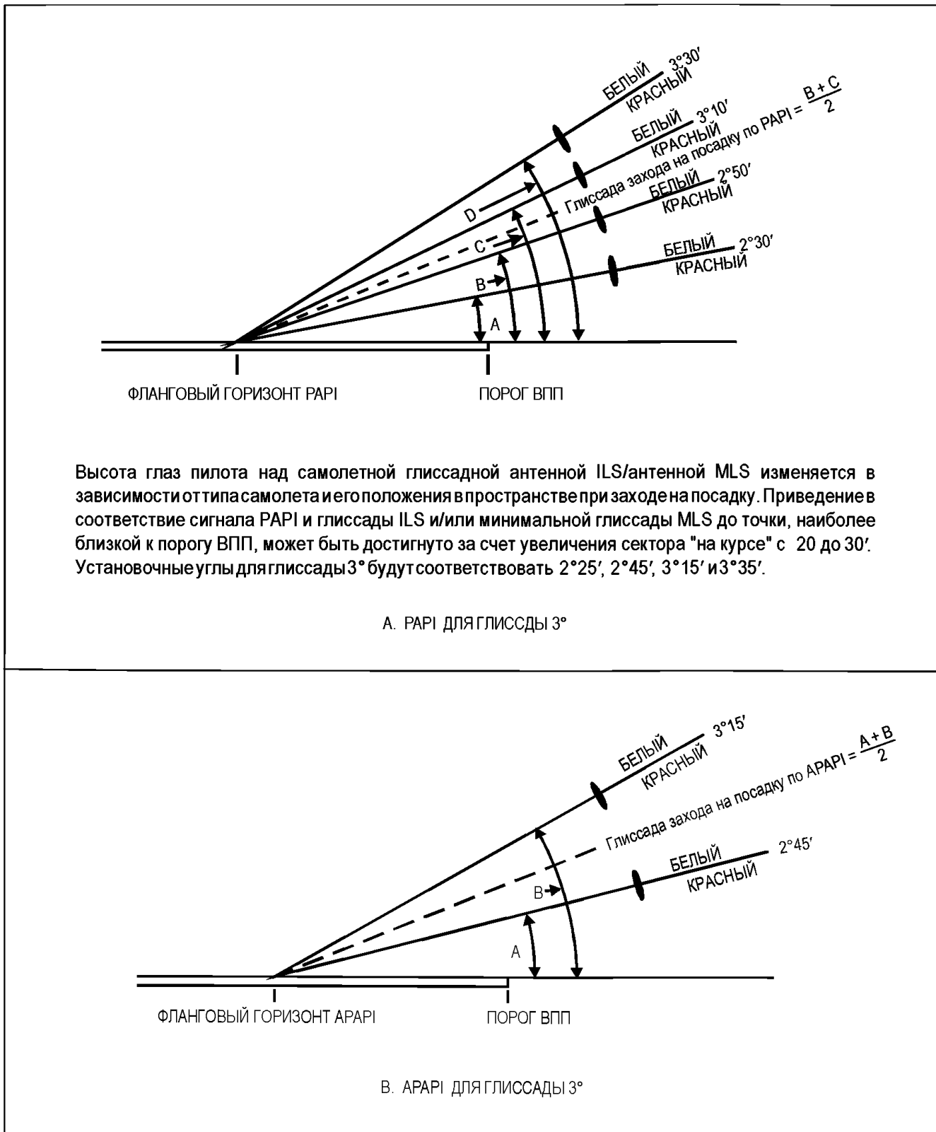
Рис. 5-20. Световые лучи и установка углов возвышения PAR1 и APAR1
