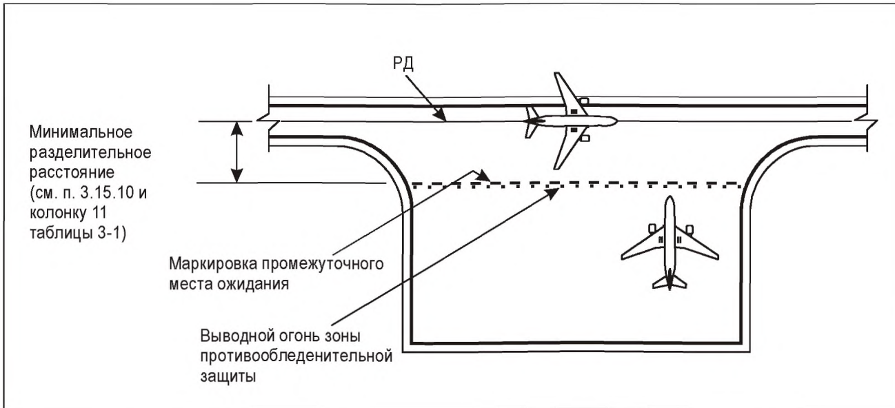
Рис. 5-28. Типичная удаленная зона противообледенительной защиты
