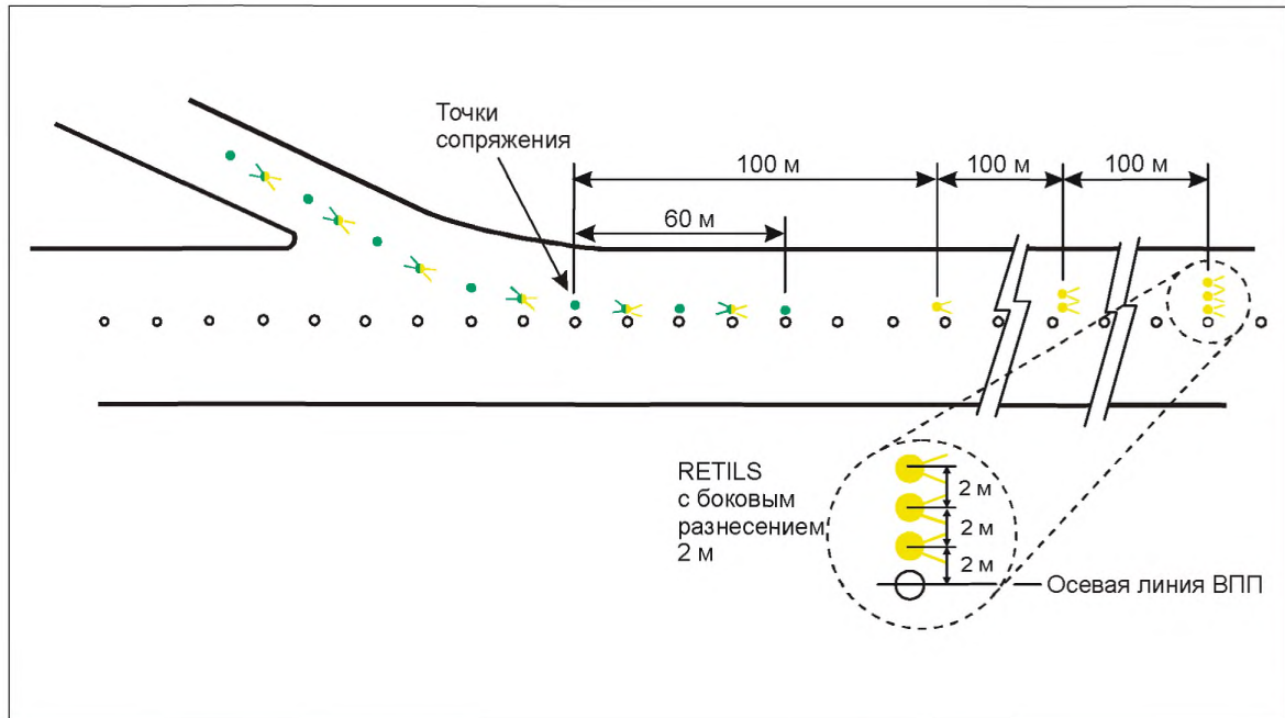
Рис. 5-25. Огни указателя скоростной выводной РД (RETILS)
