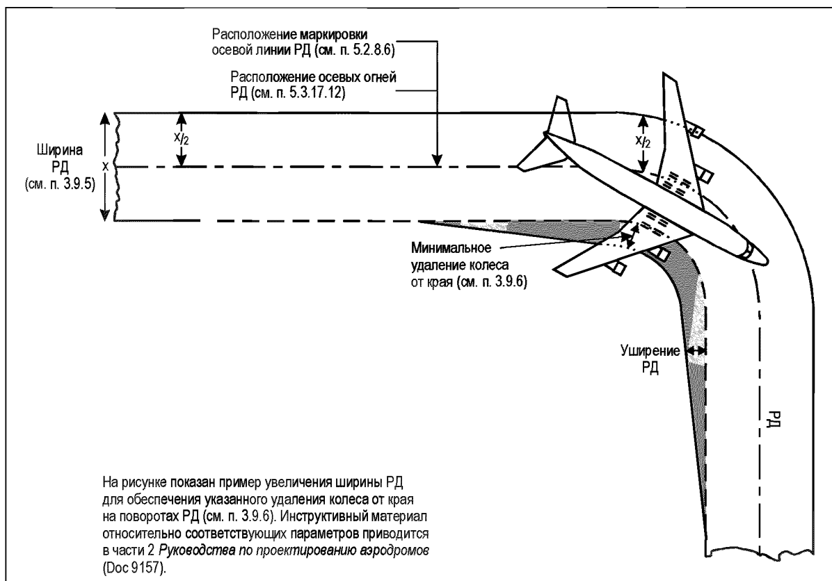
Рис. 3-2. Поворот РД
