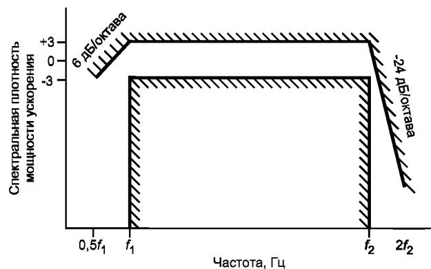
Рисунок 2 — Границы допуска для спектральной плотности мощности ускорения
