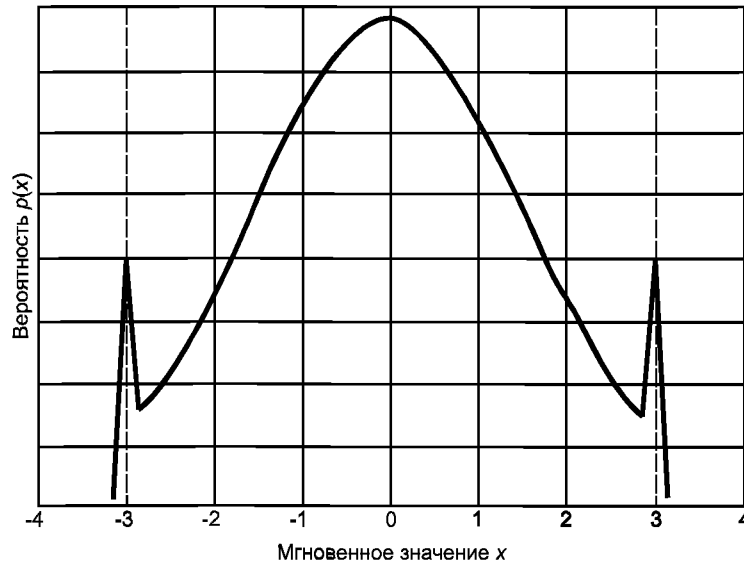
Рисунок А.3 — Негассовская плотность вероятности распределения
