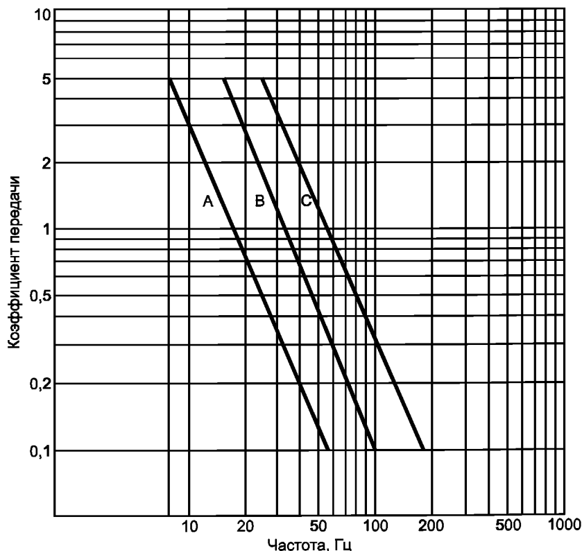
Рисунок А.6 — Коэффициент передачи виброизолятора
