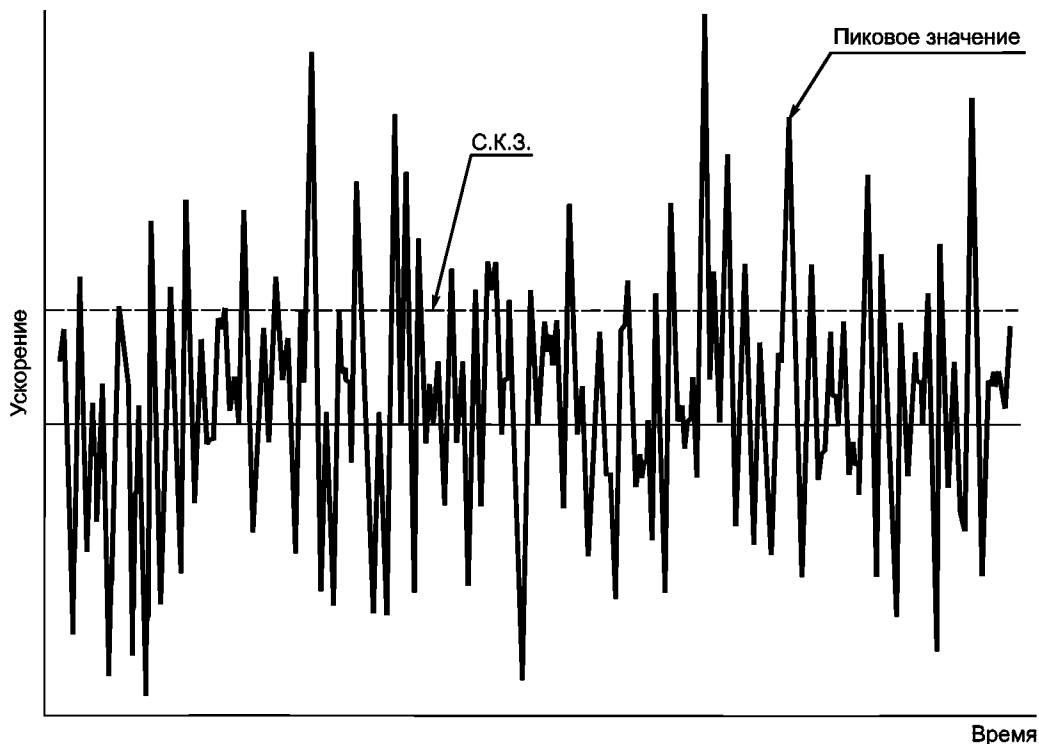
Рисунок А.2 — Отсечка (ограничение) сигнала
