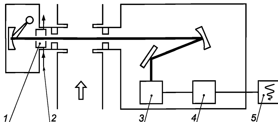
1 — кювета для калибровочных газовых смесей; 2 — ввод для калибровочных газовых смесей; 3 — приемник оптического излучения; 4 — блок электронной обработки данных; 5 — регистратор данных
