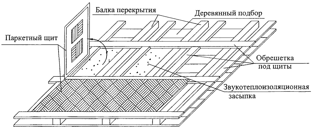
Рисунок 2 - Схема разборки чистых полов и лаг
