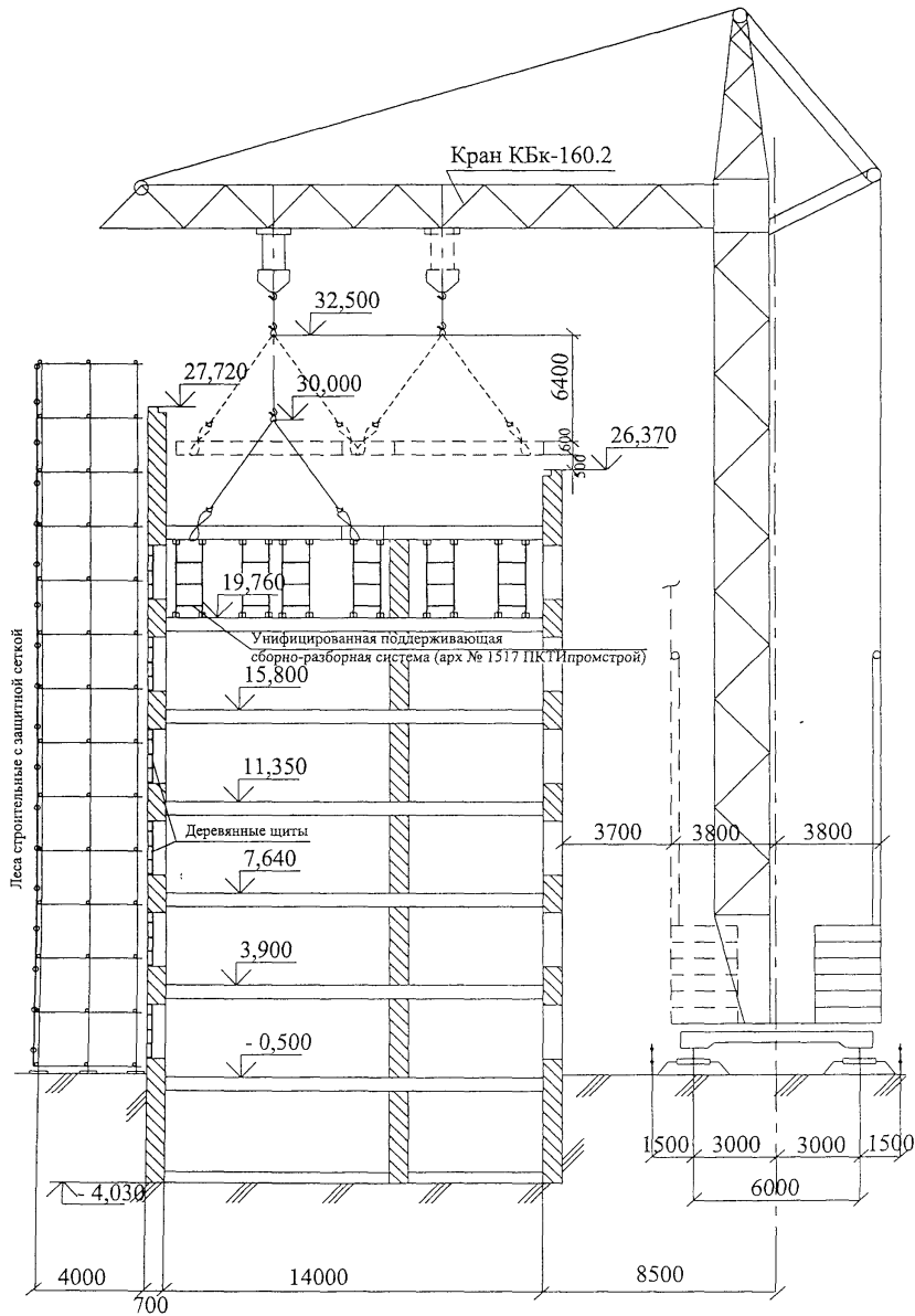
Рисунок 5 - Схема привязки крана на период разборки перекрытий.
