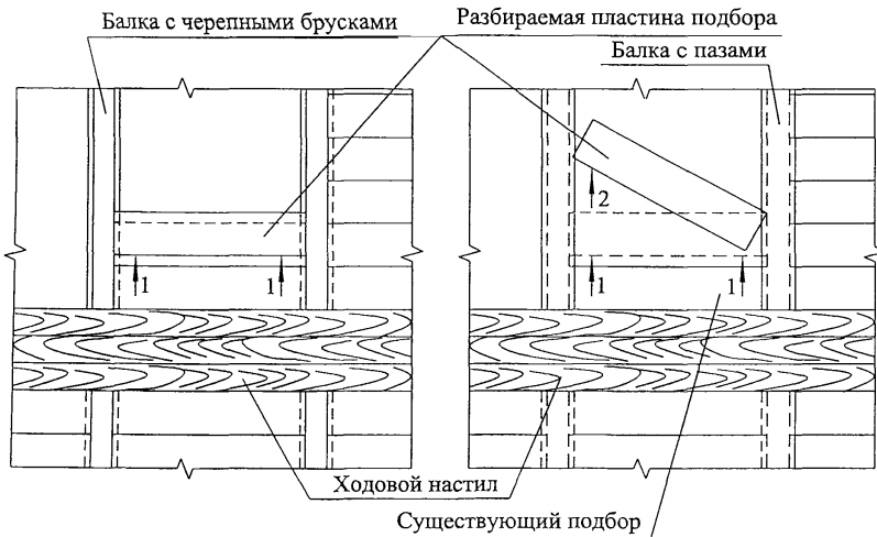
Рисунок 4 - Схема разборки деревянного подбора
