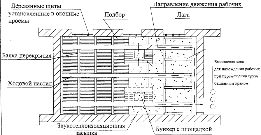
Рисунок 3 - Схема удаления звукотеплоизоляции (засыпки) перекрытия
