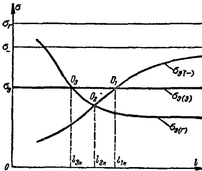
Рис. 2. Кривые зависимости напряжения провода от длины пролета при расчете провода по тем исходным условиям для случая l_{1к} > l_{2к} > l_{3к} .
