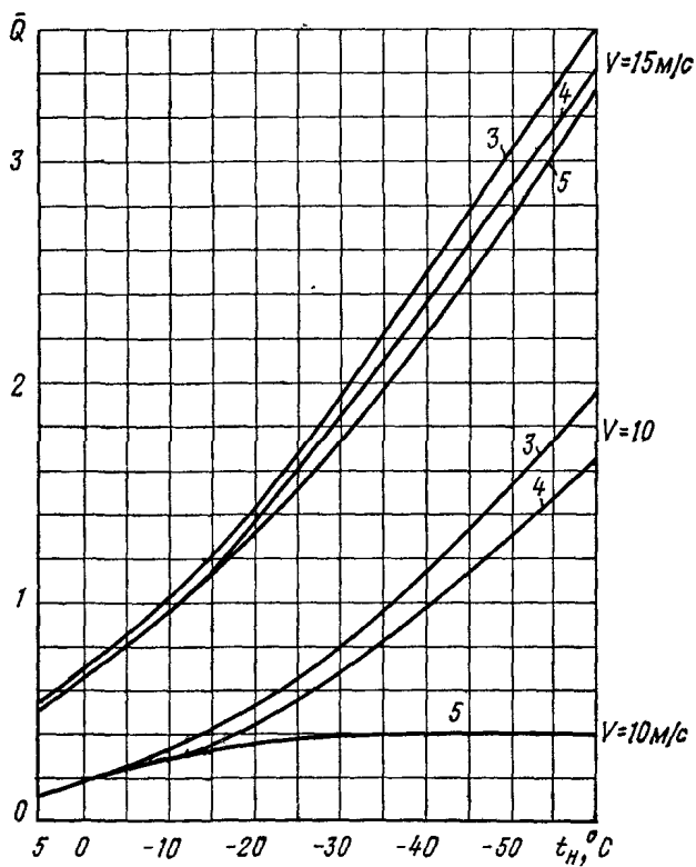
Рис. 8. Величина относительных теплотерь ( \bar{Q} ) для помещений 3—5-го этажей шестиэтажного здания с избыточным притоком в рабочее время
