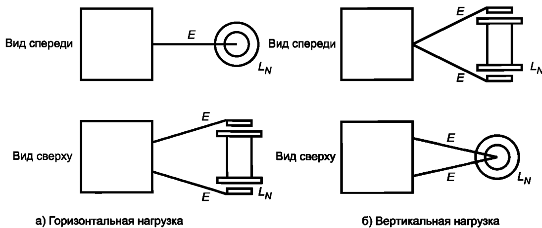
Рисунок 2 — Минимальные размеры металлической пластины заземления
