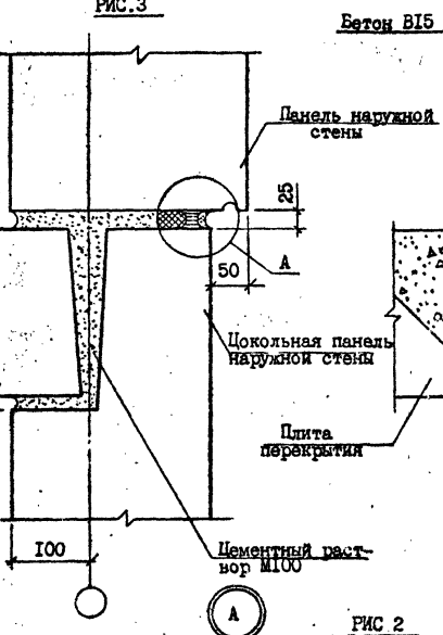
ВАРИАНТ ЗАДЕЛКИ СТЫКА ВУЛКАНИЗИРУЮЩЕЙ МАСТИКОЙ
