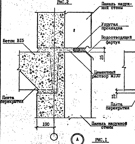
ВАРИАНТ ЗАДЕЛКИ СТЫКА НЕТВЕРДЕЮЩЕЙ МАСТИКОЙ
