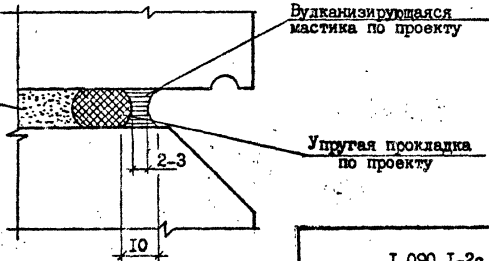
ВАРИАНТ ЗАДЕЛКИ СТЫКА ВУЛКАНИЗИРУЮЩЕЙ МАСТИКОЙ
