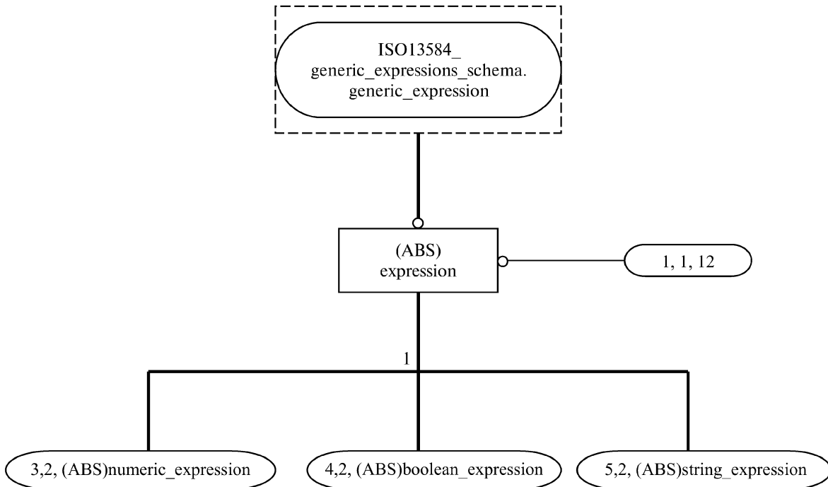
Рисунок С.2 — ISO13584_expressions_schema — EXPRESS-G диаграмма 1 из 12. Строковая типизация выражений
