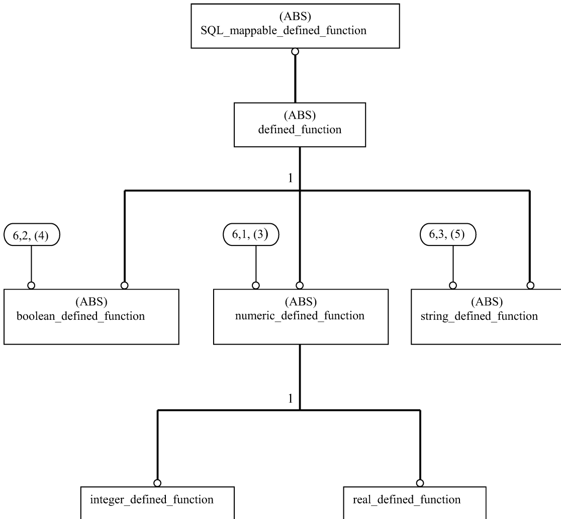
Рисунок С.7 — ISO13584_expressions_schema — EXPRESS-G диаграмма 6 из 12. defined_function
