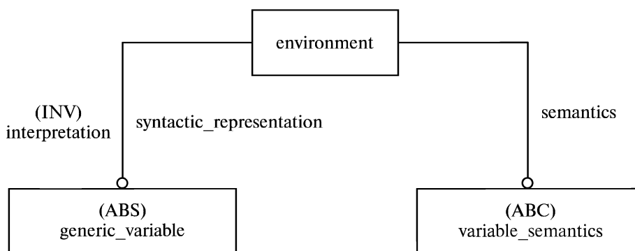
Рисунок D.1 — Связь синтаксиса и семантики переменной
