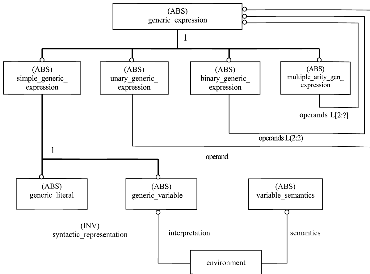
Рисунок С.1 — ISO13584_generic_expressions_schema — EXPRESS-G диаграмма 1 из 1
