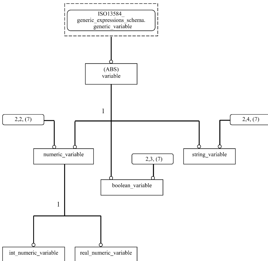
Рисунок С.3 — ISO13584_expressions_schema — EXPRESS-G диаграмма 2 из 12. Переменные
