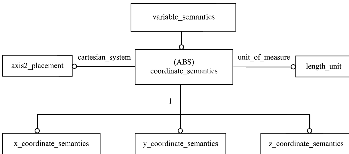
Рисунок D.4 — Пример определения понятия, не представленного в модели: координаты
