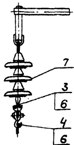
Рис. 3 Три провода (остальное см. рис. 1)
