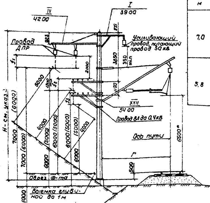
Схема 29 однопутная учасок
