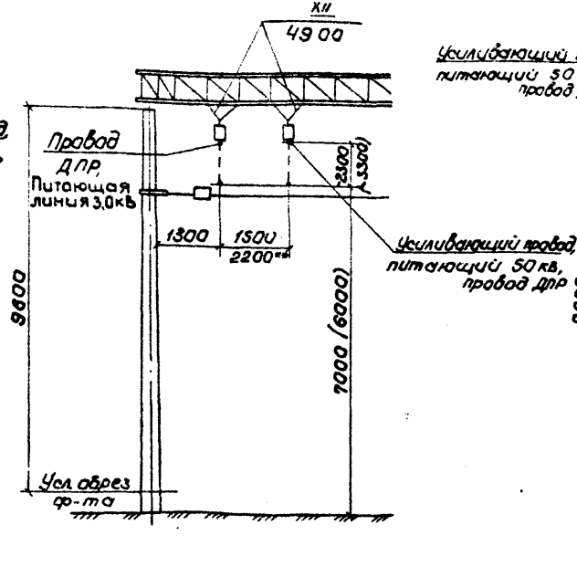
Схема 49 Двухпутный и однопутный участок
