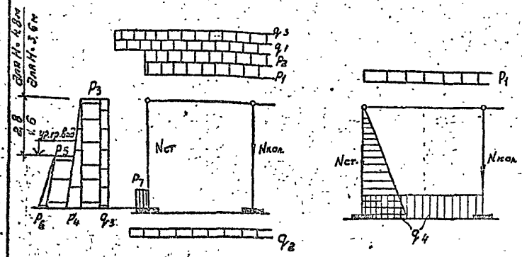
Рис. 1. Схемы расчетных сочетаний нагрузок.
