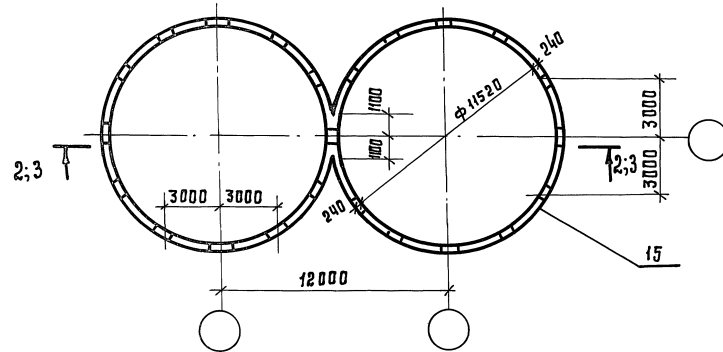
Схема расположения стен
