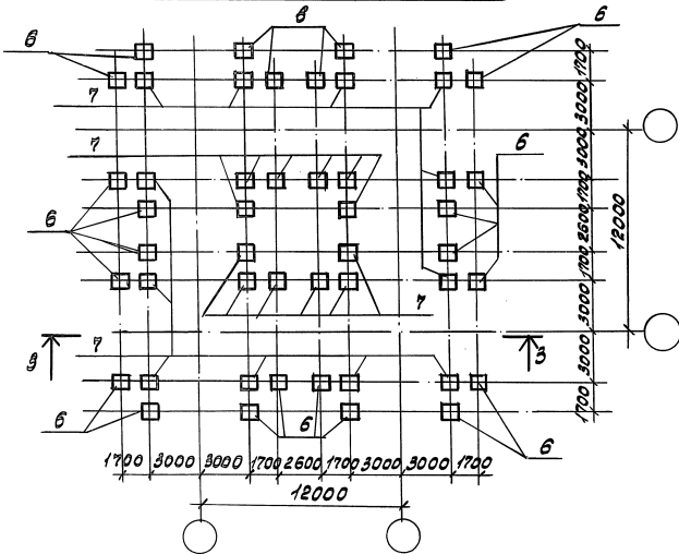
Силосный корпус 4-12-108-300 Схема расположения плиты днища.
