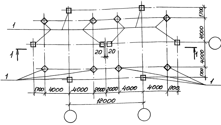
Силосный корпус 2-12-108-300 в. Схема расположения колонн
