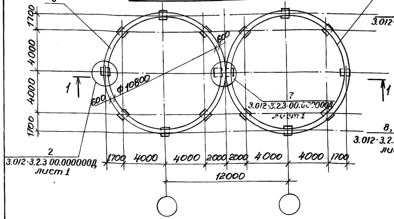
Силосный корпус 2-12-108-300 в. Схема расположения стен
