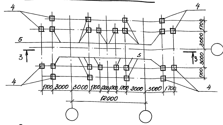
Силосные корпуса 2-12-108-180, 2-12-108-300. Схема расположения плиты днища
