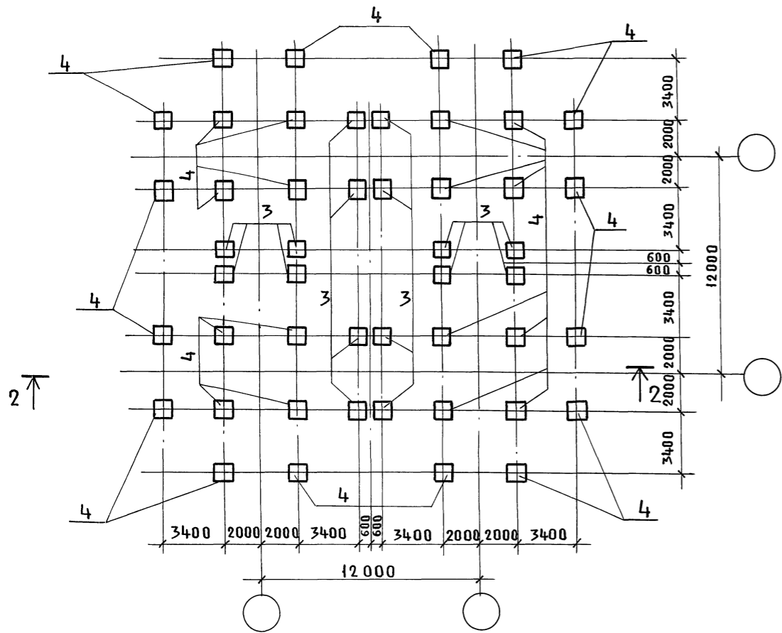
Силосный корпус 4-12-60-300 Схема расположения плиты дна
