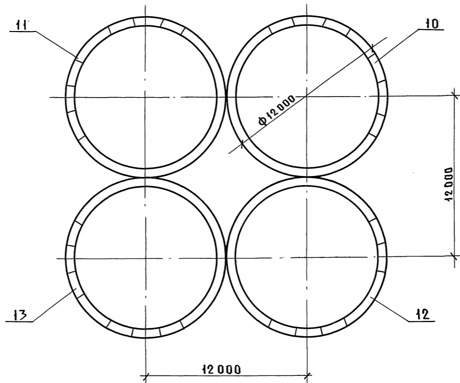
Схема расположения втулок в балках дна
