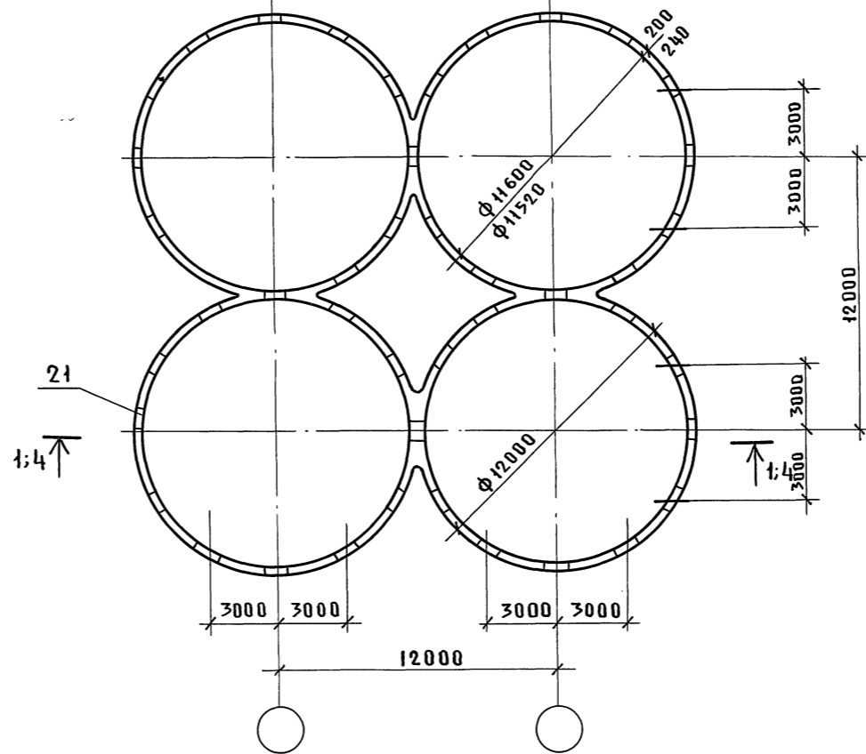
Силосный корпус 4-12-60-300
