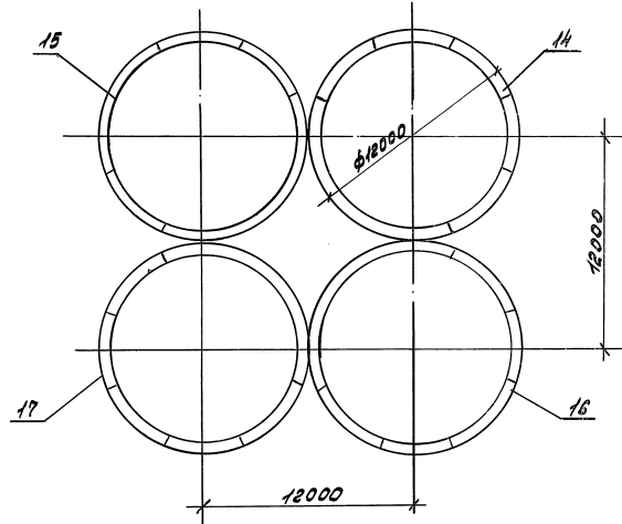
Силосные корпуса 4-12-60-300, 4-12-108-300, 4-12-108-300В, 4-12-144-264В. Схема расположения плит набысиасного перекрытия.
