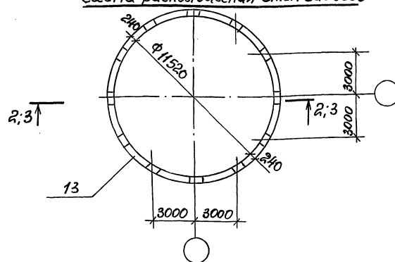
Схема расположения стен силосов
