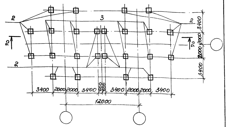
Силосные корпуса 2-12-60-180, 2-12-60-300 Схема расположения плиты днища
