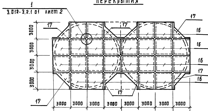
Схема расположения плит надсилосного перекрытия
