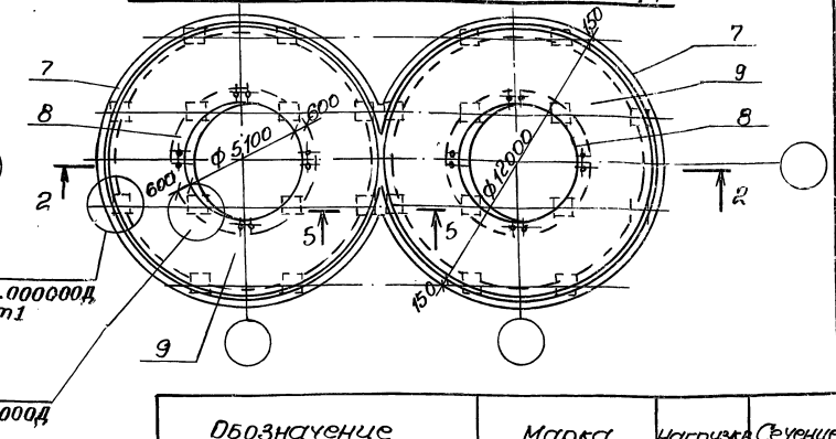
Силосные корпуса 2-12-60-180, 2-12-60-300 Схема расположения плиты днища
