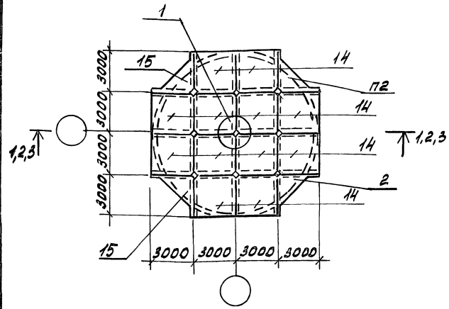
Схема расположения плит надсилосного перекрытия
