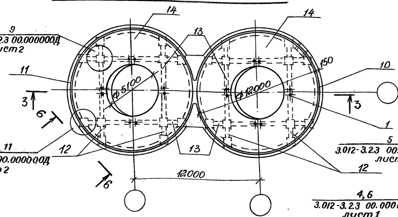
Силосные корпуса 2-12-108-180, 2-12-108-300. Схема расположения плиты днища
