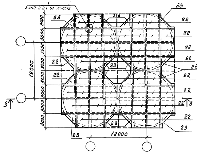
Силосные корпуса 4-12-60-300, 4-12-108-300, 4-12-108-300В, 4-12-144-264В. Схема расположения плит набысиасного перекрытия.
