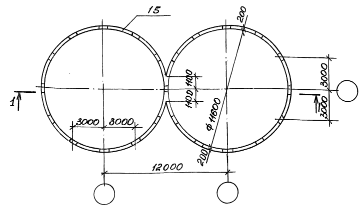
Силосный корпус 2-12-108-300 в. Схема расположения стен
