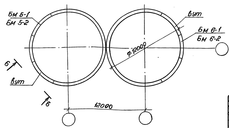
Силосный корпус 2-12-108-300 Схема расположения втулок в балках днища
