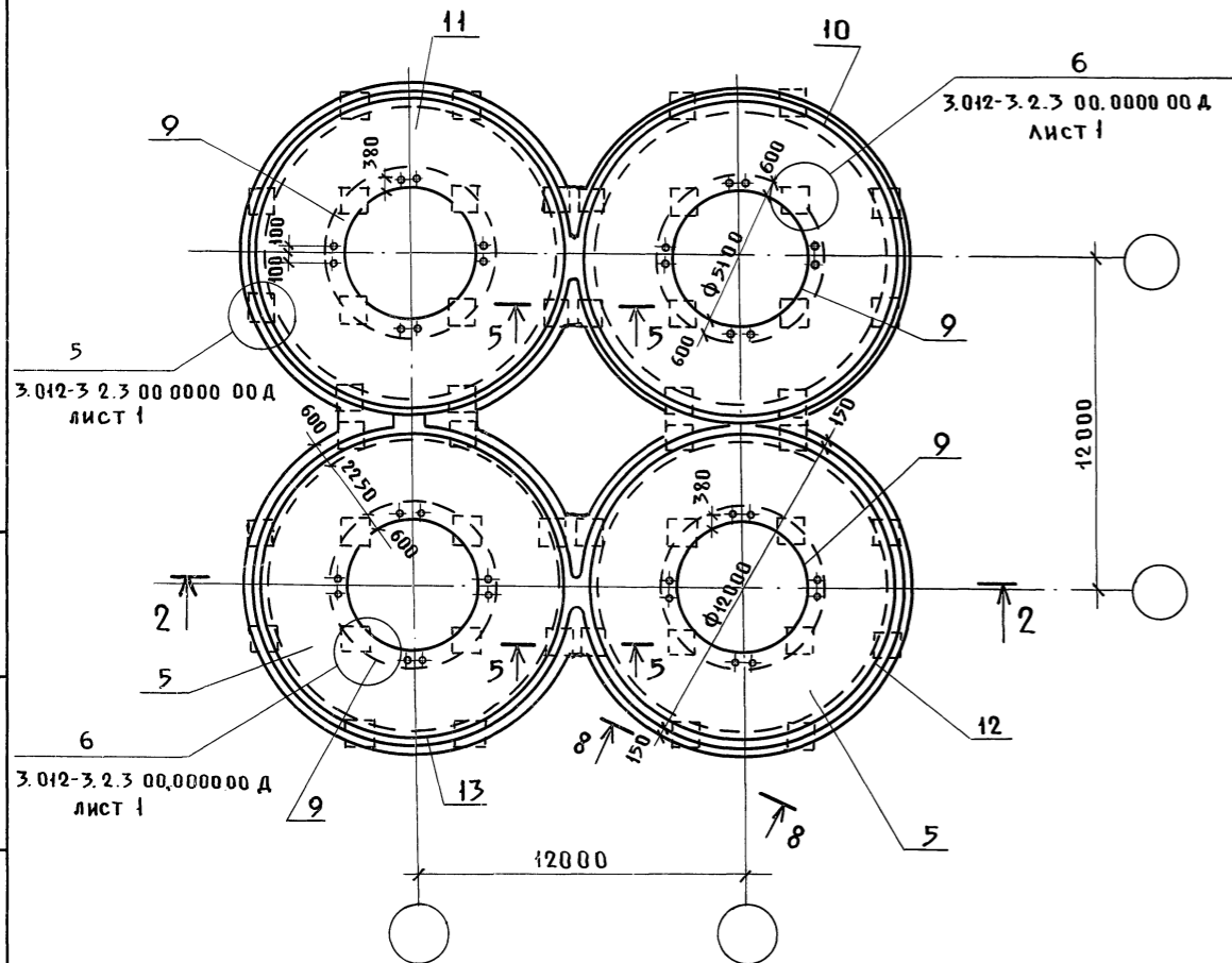
Силосный корпус 4-12-60-300 Схема расположения плиты дна
