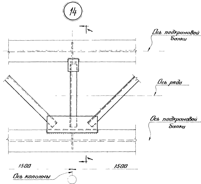
По 1-1
