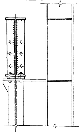
По 1-1
