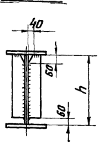
По 1-1
