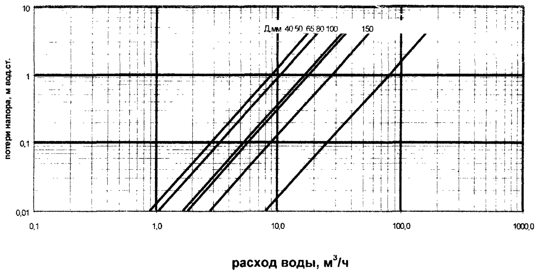
потери напора в турбинных счетчиках воды
