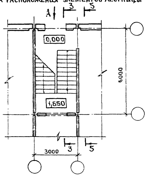
СХЕМА РАСПОЛОЖЕНИЯ ЭЛЕМЕНТОВ ЛЕСТНИЦЫ
