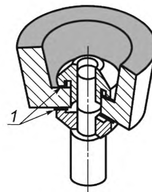
1 — прокладка
