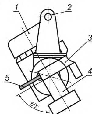
1 — двигатель; 2 — подвеска; 3 — ограждение круга; 4 — ось поворота; 5 — отрезной круг
