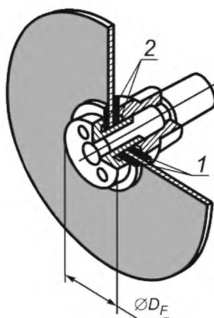
1 — прокладка; 2 — выточка
