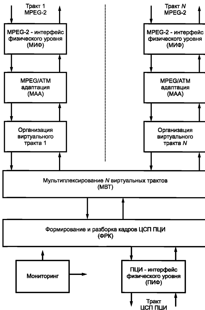
Рисунок 4.1 — Функциональная архитектура аппаратуры преобразования MPEG → ПЦИ и ПЦИ → MPEG
