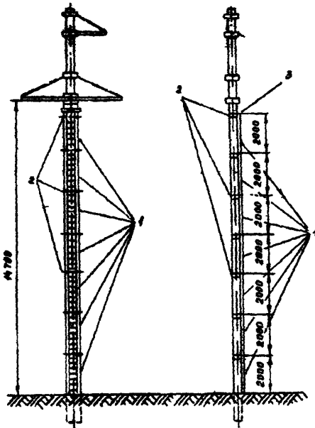
Рис. 5.4. Лестница разборная переносная: 1 - секция; 2 - хомуты для крепления черной, третьей и пятой секций (сверху) к опоре; 3 - фиксаторы
