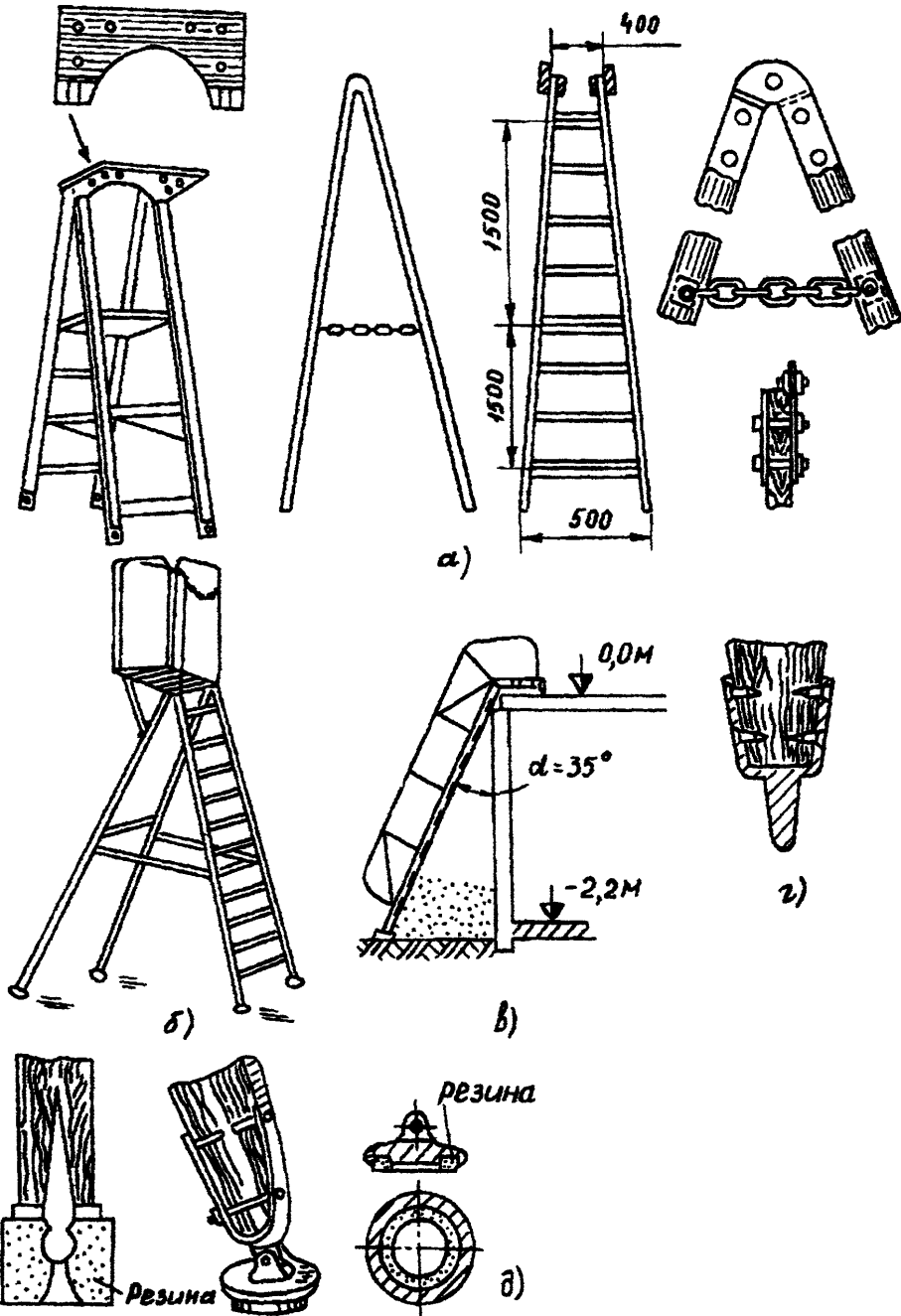
Рис. 5.3. Стремянки:
