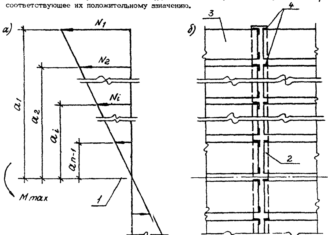
Рис. 17. Схема распределения продольных усилий в сварных соединениях плит от изгибающего момента в диске покрытия
