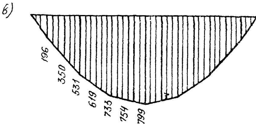
Рис. 26. К примеру расчета. Схема горизонтальных поперечных нагрузок (а), эпюры поперечных сил (б) и моментов в э диске покрытия от воздействия ветра. Нагрузки и поперечные силы в кН, моменты - в к 2 м
