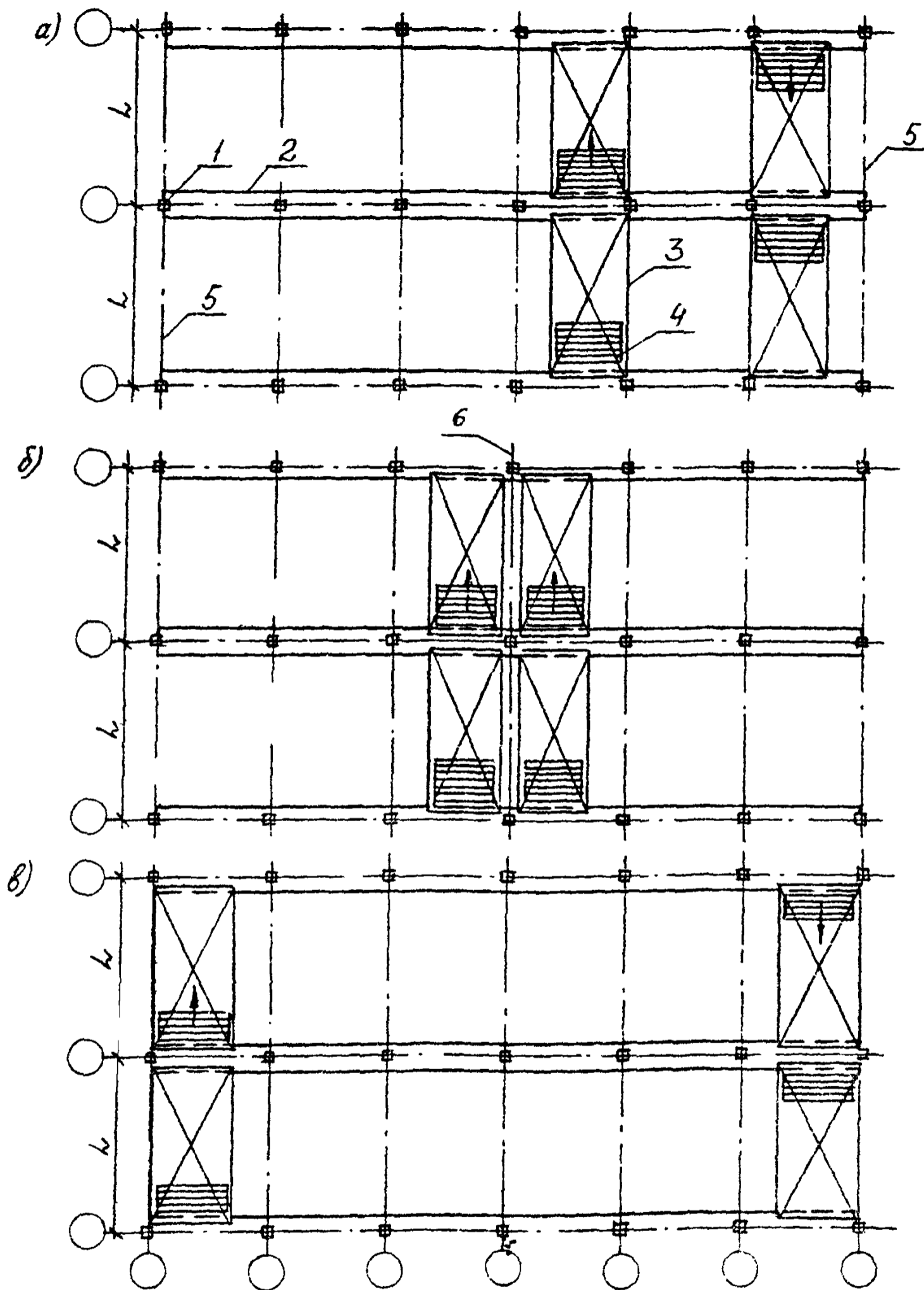
Рис.6. Схемы расположения кранов для определения усилий в диске покрытия
