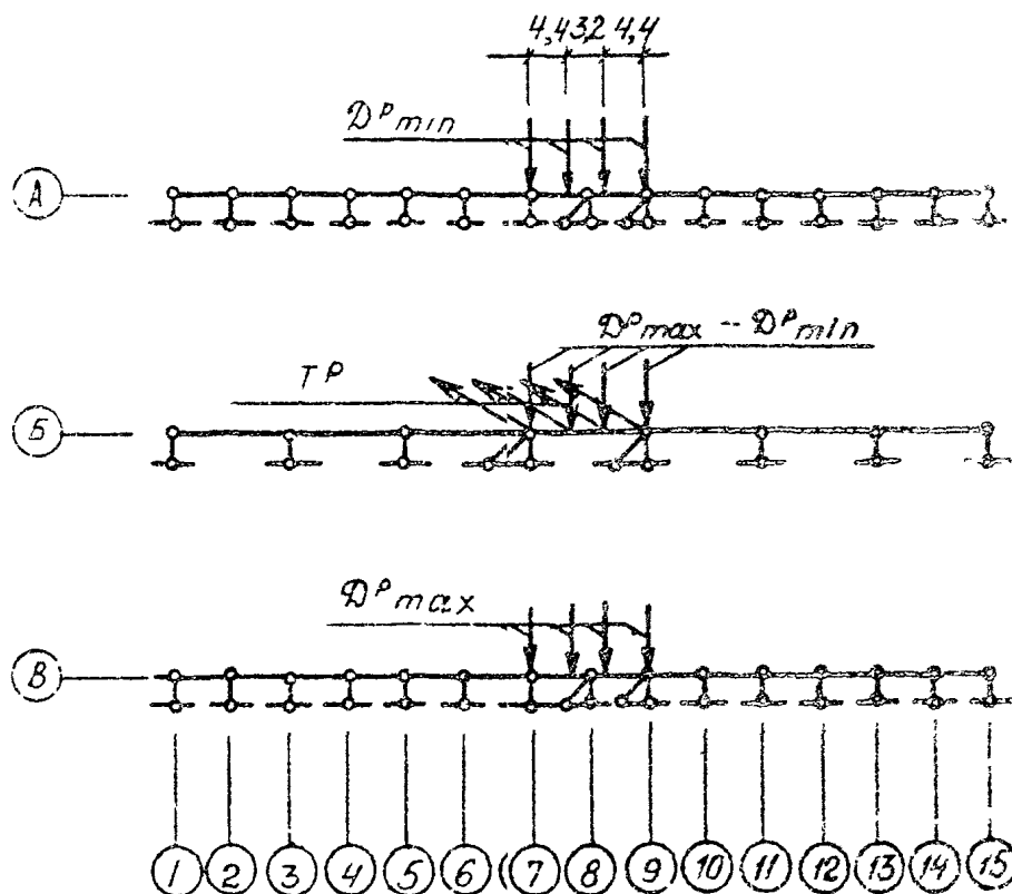
Рис. 28. К примеру расчета. Схема приложения нагрузок от колес кранов при определении изгибающих моментов в диске покрытия
