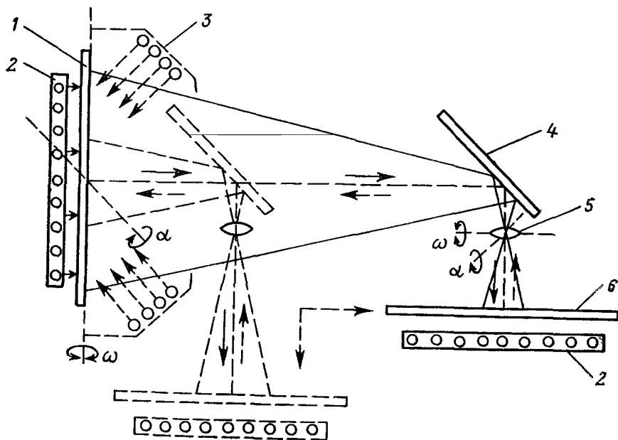
Рис. 6.1. Принцип проектирования
