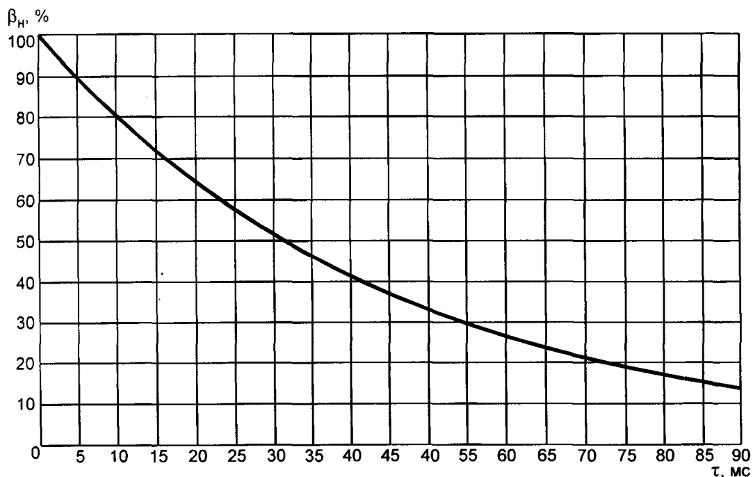
Рисунок 3 — Содержание аperiodической составляющей в процентах
