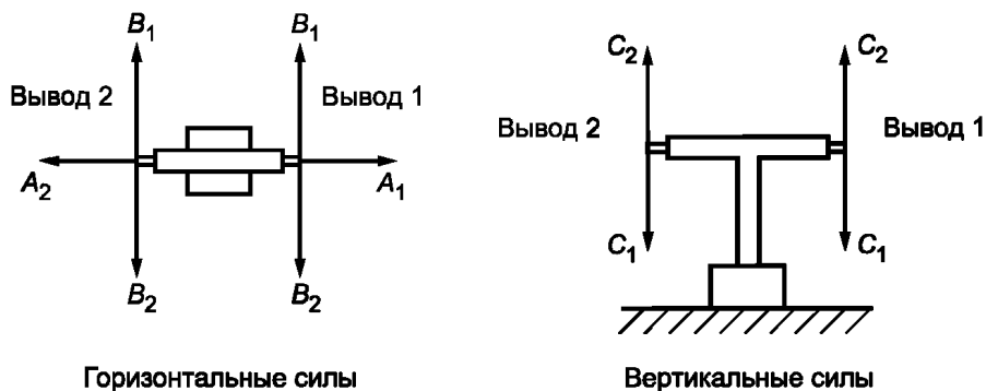
а) Статические нагрузки на выключатель
