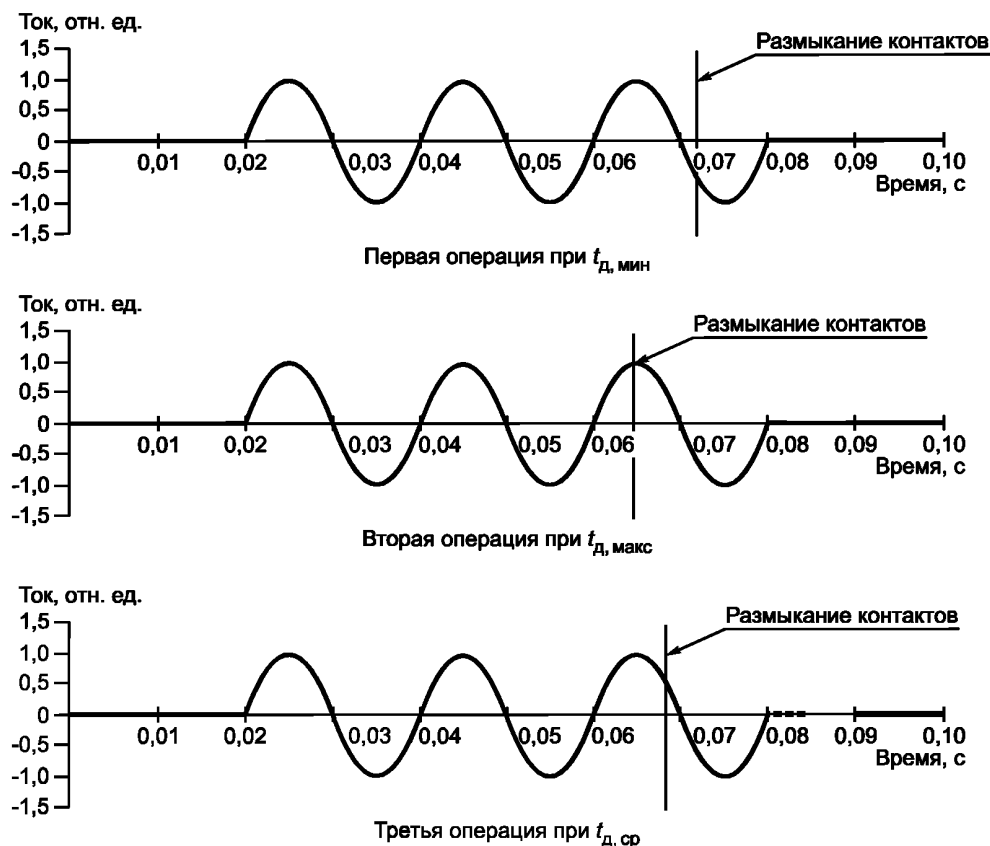
Рисунок 11 — Регулирование момента размыкания контактов относительно фазы тока при однополюсном отключении симметричного тока в режимах Т10, Т30, Т60, Т100s, Тcr1, Тcr2, Тcr3 выключателями с U_{ном} \leq 35 кВ
