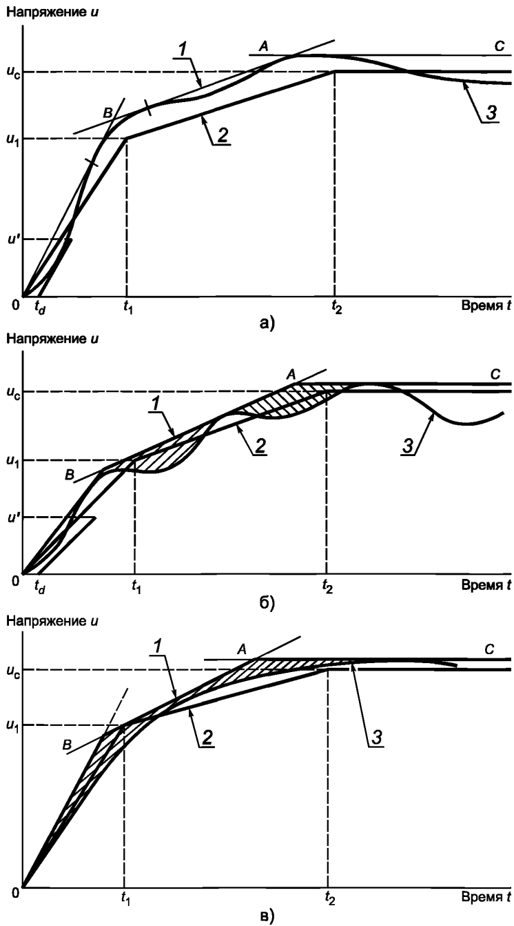
Рисунок 8 — Построение огибающей ПВН, определяемого четырьмя параметрами
