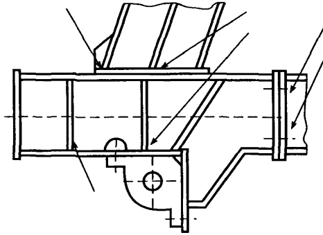
Узел крепления опоры к ходовой тележке козлового крана КДКК -10.
