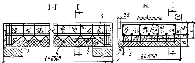
Рис. 10. Конструкция изгибаемого железобетонного элемента, нагреваемого до температуры более 400^{\circ}\text{C} со стороны растущей зоны
