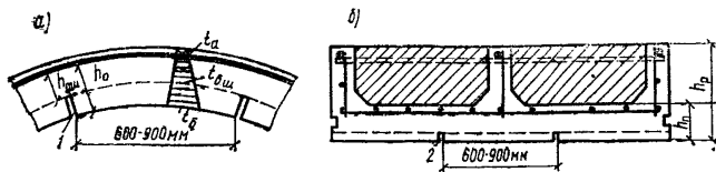
Рис. 9. Швы со стороны нагреваемой поверхности в конструкциях из жаростойкого бетона
