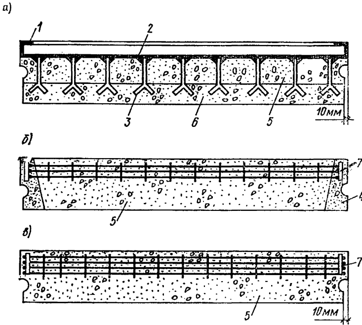
Рис. 11. Конструкции панелей из легкого жаростойкого бетона
