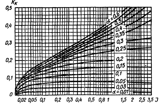
Рис. 2. Номограммы для определения коэффициентов \xi_k и K_k
