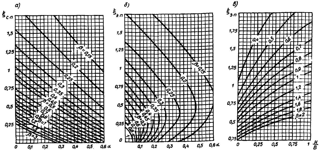
Рис. 3. Номограммы для определения коэффициентов а — \xi_{c,n} ; б — \xi_{k,n} ; в — \xi_{3,n}
