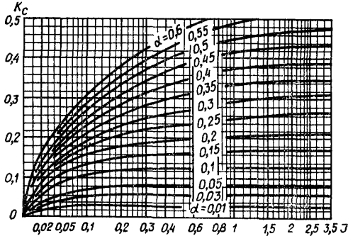
Рис. 1. Номограммы для определения коэффициентов \xi_c и K_c
