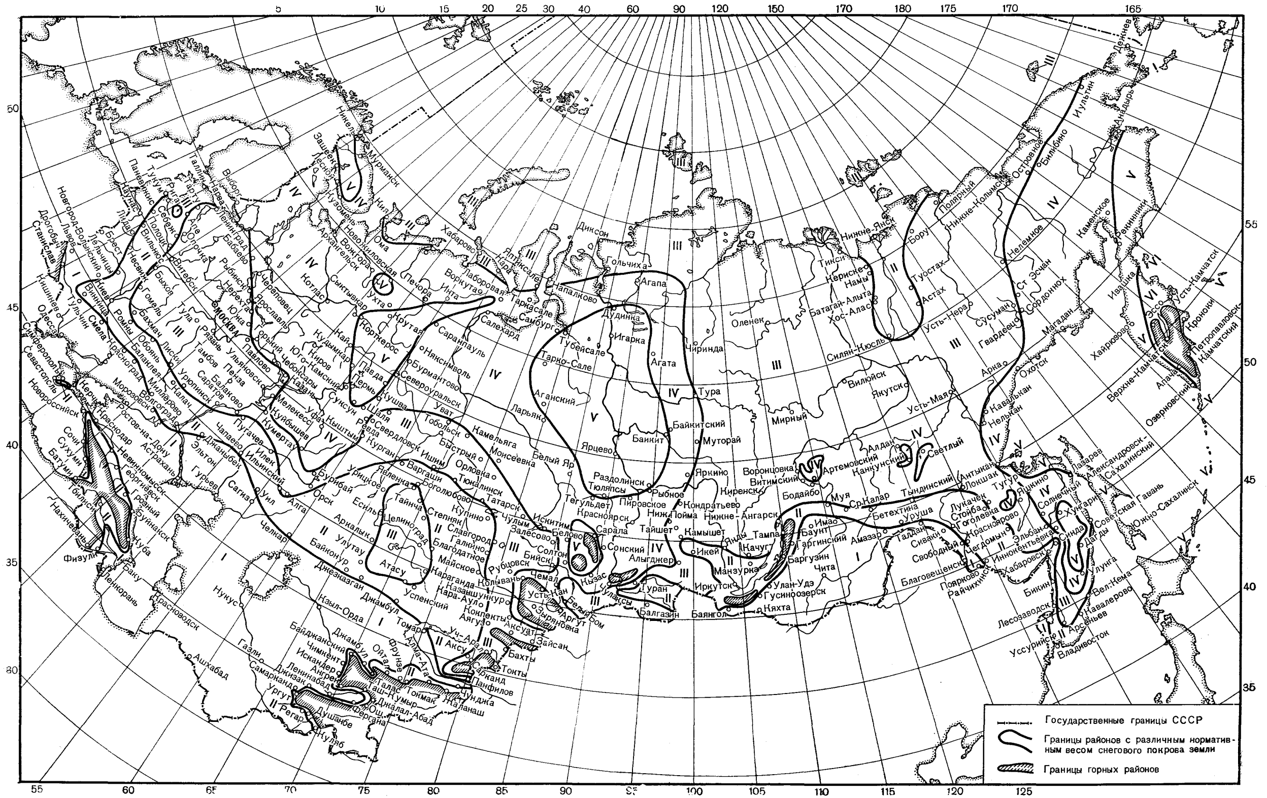
Районирование территории СССР по весу снегового покрова
