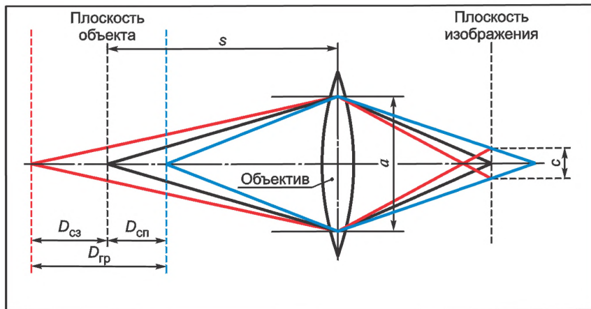
Рисунок Б.1 — Параметры для вычисления глубины поля
