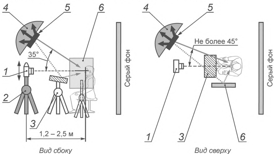
Рисунок Б.4 — Организация освещения фотолаборатории с использованием одного источника освещения
