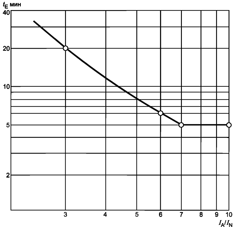
Рисунок 2 — График зависимости минимального значения времени t_E моторов от отношения пусковых токов I_A/I_N
