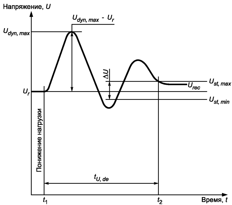
Рисунок А.2 — Характеристика переходного напряжения (понижение нагрузки)
