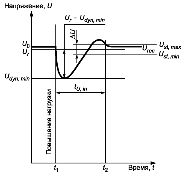
Рисунок А.1 — Характеристика переходного напряжения (повышение нагрузки)
