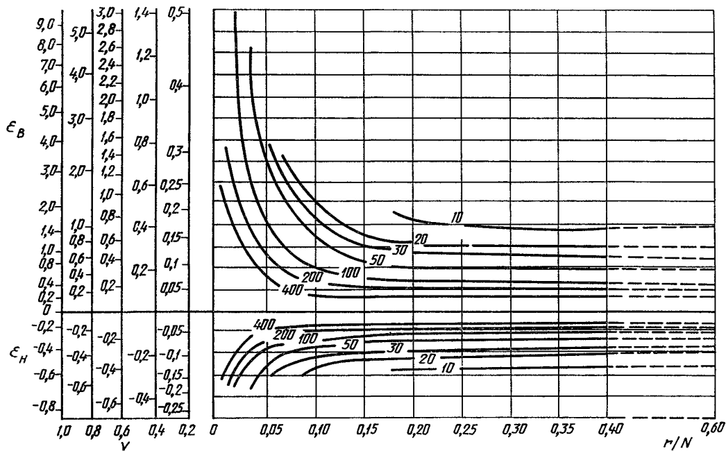
Цифры на кривых указывают объем выборки Черт. 4
