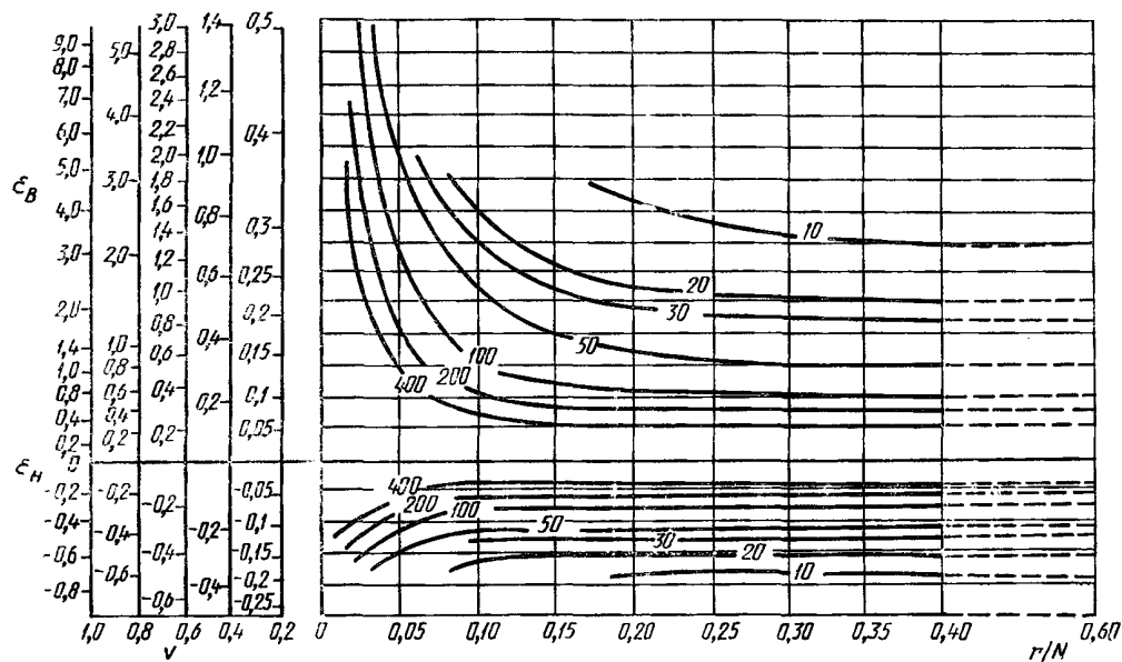
Цифры на кривых указывают объем выборки Черт. 8
